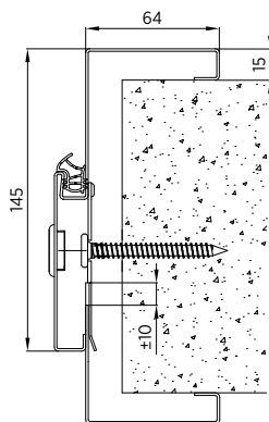
Rys. 7. Ościeżnica obejmująca – opcja
