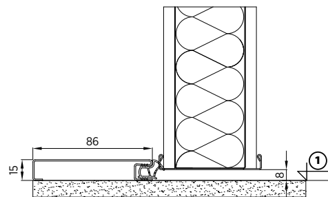
Rys. 15. Przekrój progu drewnianego – rozwiązanie standardowe
