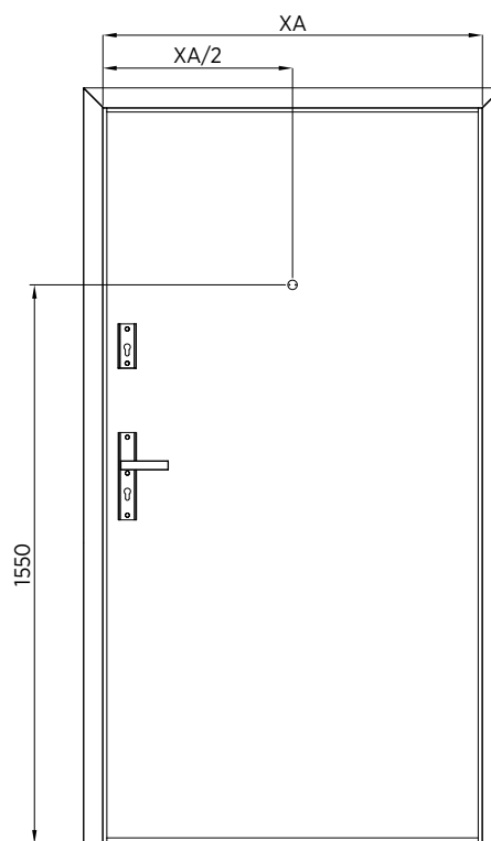
Rys. 16. Montaż wizjera panoramicznego lub elektronicznego na skrzydle
