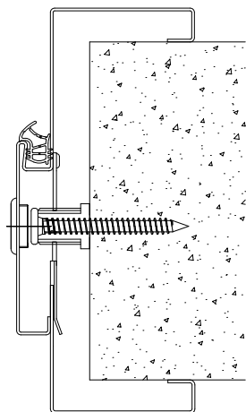
Rys. 19. Sposób montażu ościeżnicy do muru pośrednio przez element rozpierający ościeżnicę w narożach
