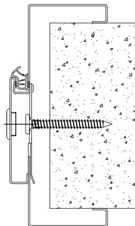
Rys. 20. Sposób montażu ościeżnicy do muru bezpośrednio przez element montażowy
