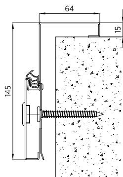
Rys. 6. Ościeżnica narożna – standard
