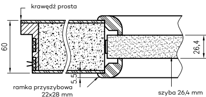
Skrzydło drzwiowe przeciwpożarowe Olimp EI60
