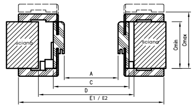
Przekrój poziomy ORB
