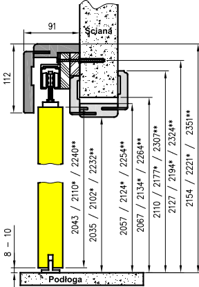
NT - przekrój pionowy na tunelu z kąt. 63 mm
