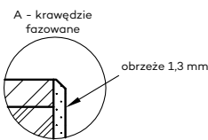
Przekrój ramienia skrzydła bezprzylgowego
