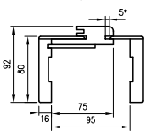
Przekrój ORB 075
