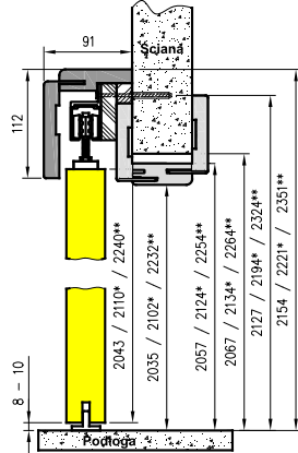
NT - przekrój pionowy na tunelu z kąt. 80 mm
