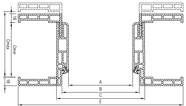
Szerokość ościeżnicy drzwi jednoskrzydowych przylgowych
