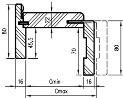
Profil ościeżnicy
