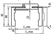
Przekrój ORB 075
