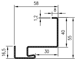
Profil ościeżnicy OSMK
