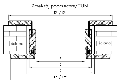
Przekrój TUN z kąt. T80
