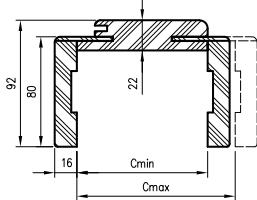
Przekrój OR/ORC z kąt. T80
