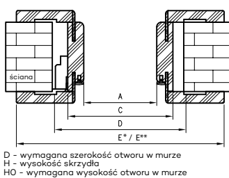
Przekrój OR z kątem T80
