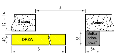
NS - przekrój poziomy (system lewy)
