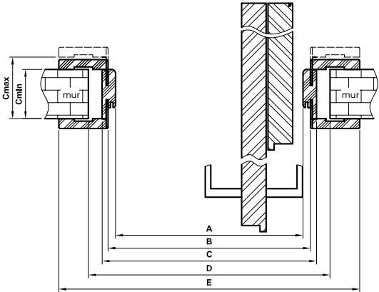
Przekrój poprzeczny drzwi składanych w pozycji otwartej*
