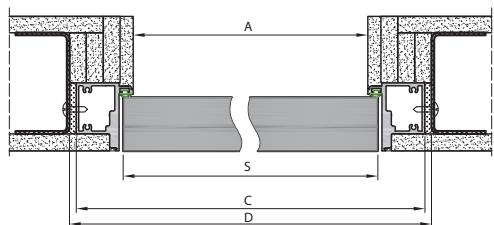
Przekrój poprzeczny drzwi Sara Eco 2 (montaż w ścianie G-K)
