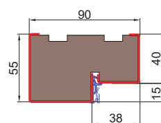
OŚCIEŻNICA DREWNIANA DO DRZWI ACERO 55
