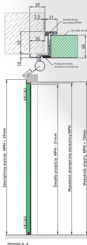
WYMIARY OŚCIEŻNICY KĄTOWEJ (TYP STD):
