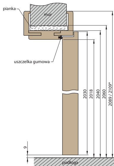
KĄTOWNIK RUCHOMY OŚCIEŻNICY Z PRZEDŁUŻONYM PIÓREM O 2CM
