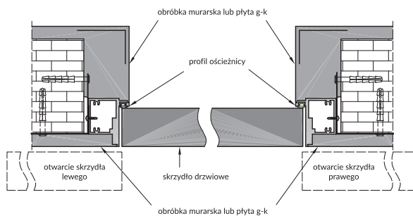
Przekrój poprzeczny drzwi Sara Eco 2 (montaż w ścianie G-K)
