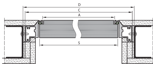
Przekrój poprzeczny drzwi Sara Eco 2 (montaż w ścianie G-K)
