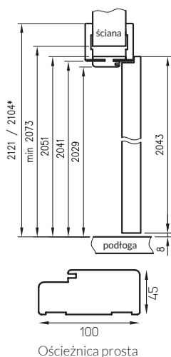
Przekrój pionowy drzwi przylgowych z OR
