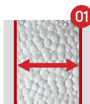
01 Skrzydło o grubości 72 mm z czterostronną przylgą, wykonane z ocynkowanej blachy laminowanej o grubości 0,6 mm, wypełnione polistyrenem spienionym
