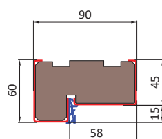
OŚCIEŻNICA DREWNIANA DO DRZWI ACERO 85
