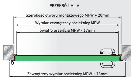
WYMIARY OŚCIEŻNICY KĄTOWEJ (TYP STD):
