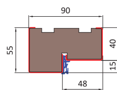
OŚCIEŻNICA DREWNIANA DO DRZWI ACERO 72
