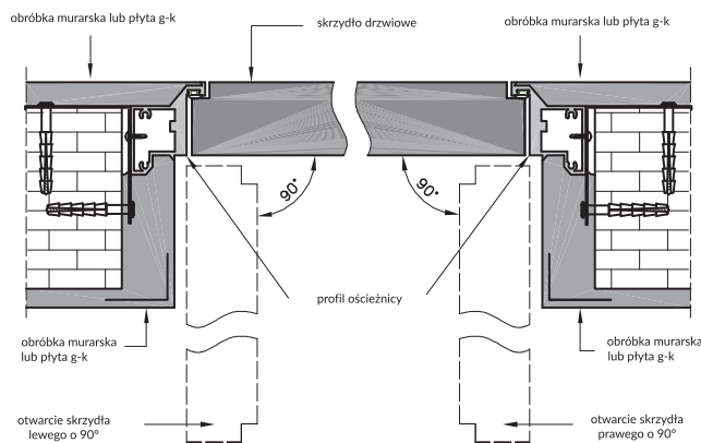
Przekrój poprzeczny drzwi Sara Eco 2 (montaż w ścianie G-K)
