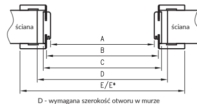
Przekrój poziomy OR
