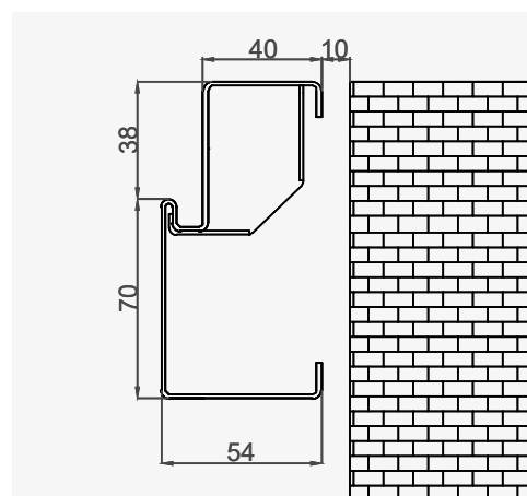
WYMIAROWANIE OŚCIEŻNICY
