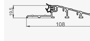
WYMIAROWANIE PROGU
