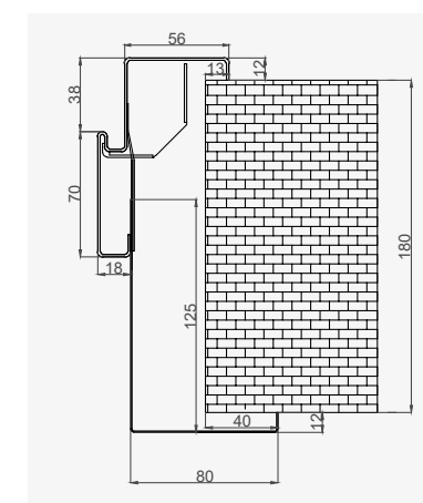
WYMIAROWANIE OŚCIEŻNICY
