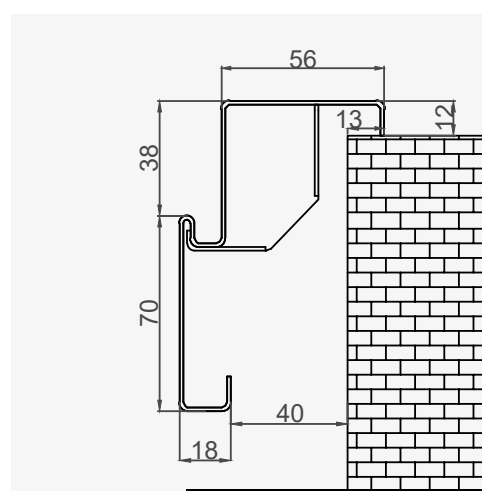
WYMIAROWANIE OŚCIEŻNICY
