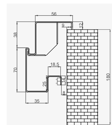
WYMIAROWANIE OŚCIEŻNICY
