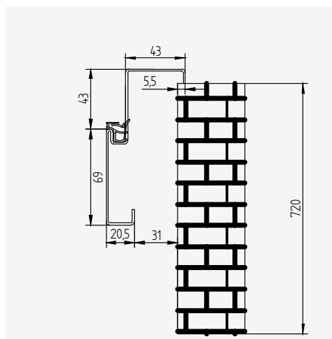
WYMIAROWANIE OŚCIEŻNICY
