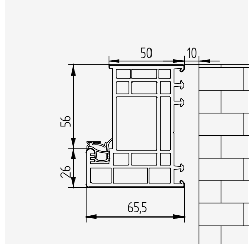
WYMIAROWANIE OŚCIEŻNICY
