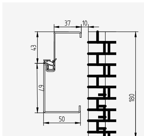
WYMIAROWANIE OŚCIEŻNICY
