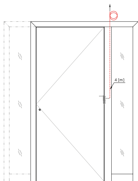
Rys. 58. Wyprowadzenie przewodu zasilającego (sterującego) z ościeżnicy dla drzwi z doświetlaniem bocznym od strony zawiasów
