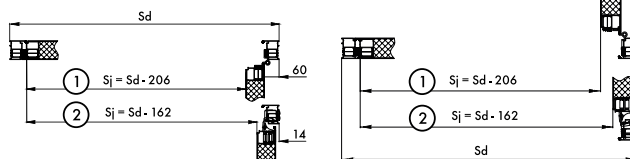
Zależności światła przejścia dla drzwi CREO
