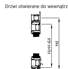
Rys. 47. Światła przejścia Hj dla drzwi DECO Basic z doświetlem górnym
