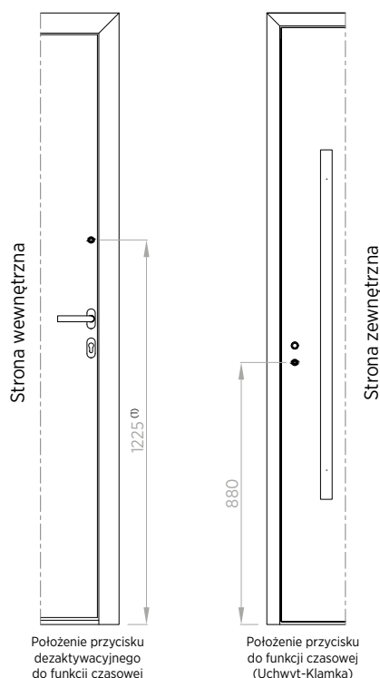
Rys. 60. Schemat położenia przycisków funkcji czasowej
