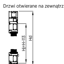
Rys. 46. Światła przejścia Hj dla drzwi DECO Basic z doświetlem bocznym
