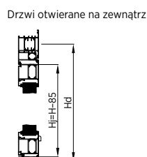
Rys. 47. Światła przejścia Hj dla drzwi DECO Basic z doświetlem górnym
