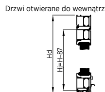
Rys. 42. Światła przejścia Hj dla drzwi DECO Basic bez doświetli
