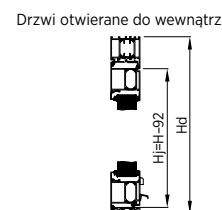
Rys. 46. Światła przejścia Hj dla drzwi DECO Basic z doświetlem bocznym
