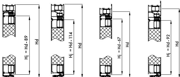
Rys. 100. Światła przejścia H j dla drzwi CREO z doświetleniem górnym
