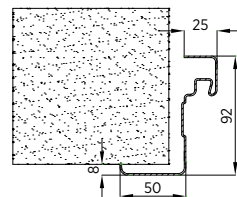
Rys. 6. Ościeżnica narożna – standard
