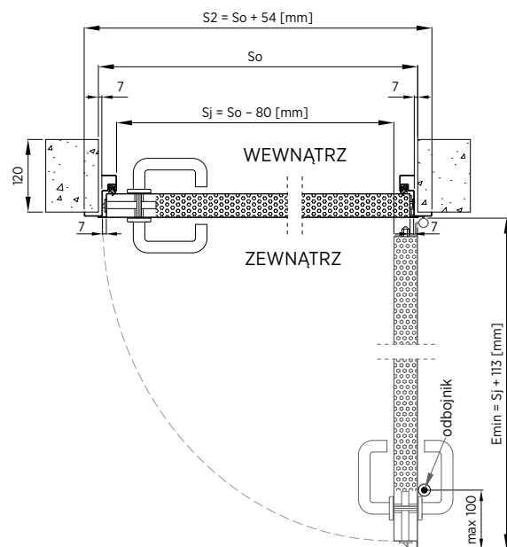
Rys. 18. Montaż drzwi jednoskrzydłowych z ościeżnicą narożną - przekrój poziomy
