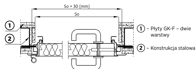
Rys. 40. Montaż do konstrukcji stalowej drzwi jednoskrzydłowych z ościeżnicą narożną - przekrój poziomy
