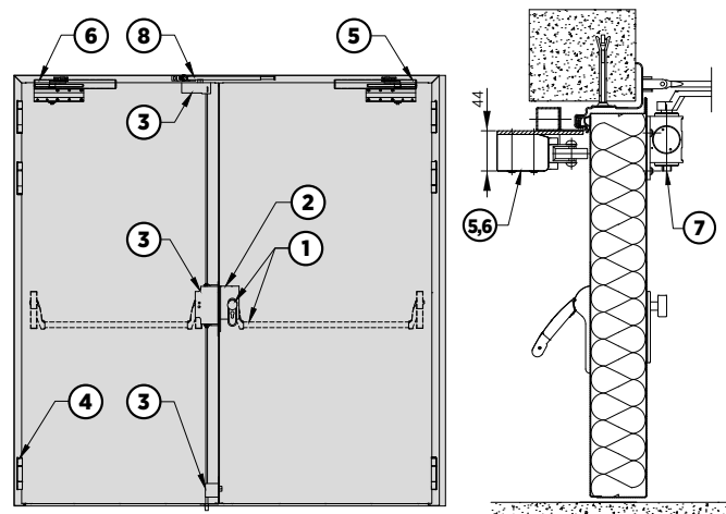
Rys. 74. Schemat układu napowietrzania drzwi stalowych płaszczone dwuskrzydłowych z funkcją paniczną – przekrój pionowy
