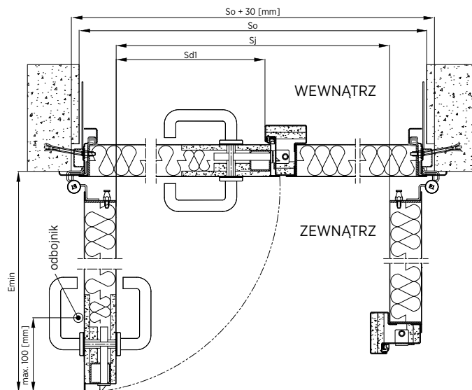
Rys. 79. Montaż na ościeżnicy narożnej drzwi dwuskrzydłowych – przekrój poziomy
