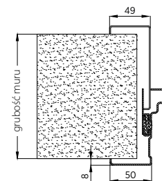
Rys. 11. Ościeżnica obejmująca z przekładką termiczną
