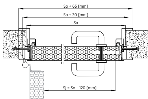
Rys. 62. Montaż do muru drzwi jednoskrzydłowych – ościeżnica obejmująca z przekładką termiczną – przekrój poziomy
