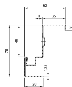
Rys. 6. Ościeżnica narożna – standard
