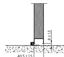
Rys. 20. Przekrój przez próg
