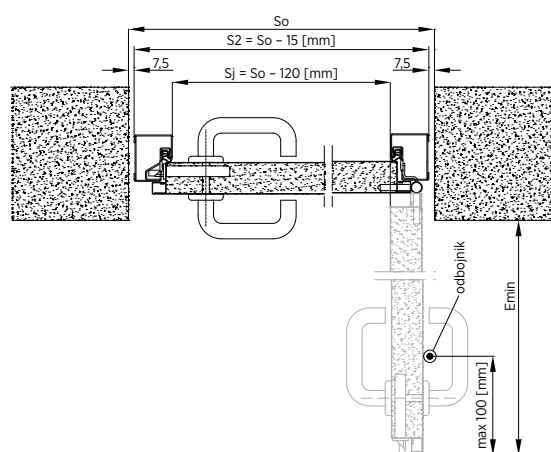
Rys. 30. Montaż drzwi jednoskrzydłowych z ościeżnicą wewnętrzną – przekrój poziomy
