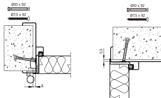
Rys. 34. Montaż ościeżnicy obejmującej, boki i nadproże drzwi jednoskrzydłowych
