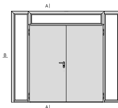
Rys. 86. Drzwi dwuskrzydłowe ECO z doświetlami bocznymi i naświetlem górnym
