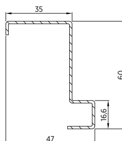
Rys. 4. Ościeżnica narożna
