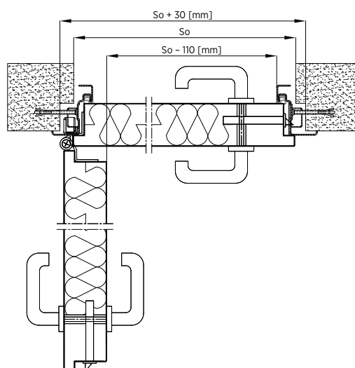
Rys. 46. Montaż do muru drzwi jednoskrzydłowych płaszczyznych ECO TECH z ościeżnicą narożną bez przekładki termicznej – przekrój poziomy
