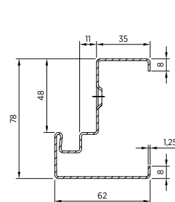
Rys. 7. Ościeżnica wewnętrzna – opcja
