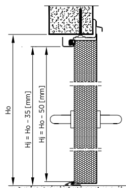
Rys. 55. Montaż do konstrukcji stalowej drzwi jednoskrzydłowych z ościeżnicą narożną bez przekładki termicznej – przekrój pionowy
