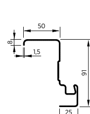
Rys. 55. Ościeżnica narożna – standard
