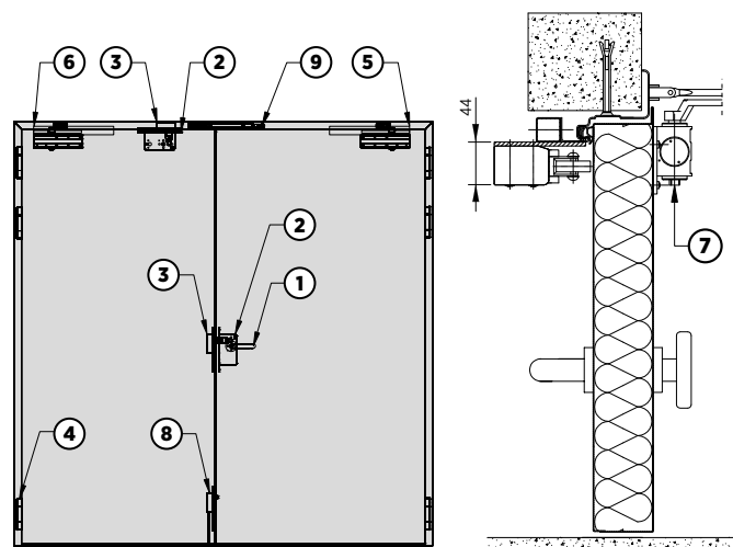
Rys. 73. Schemat drzwi dwuskrzydłowych – przekrój pionowy z układem napowietrzania
