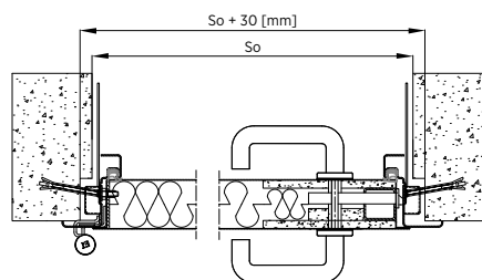
Rys. 73. Montaż do muru drzwi jednoskrzydłowych z ościeżnicą narożną – przekrój poziomy
