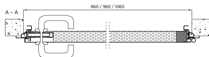
Rys. 3. Przekrój poziomy drzwi stalowych płaszczone ECO BASIC UNI z ościeżnicą narożną
