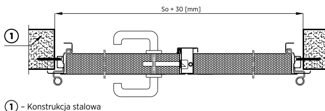
Rys. 56. Montaż do konstrukcji stalowej drzwi dwuskrzydłowych z ościeżnicą narożną bez przekładki termicznej – przekrój poziomy
