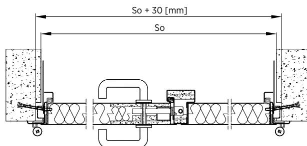
Rys. 75. Montaż do muru drzwi dwuskrzydłowych z ościeżnicą narożną – przekrój poziomy
