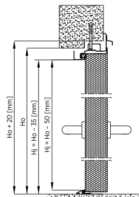
Rys. 53. Montaż do muru drzwi dwuskrzydłowych z ościeżnicą narożną bez przekładki termicznej – przekrój pionowy
