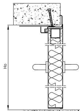
Rys. 74. Montaż do muru drzwi jednoskrzydłowych z ościeżnicą narożną – przekrój pionowy
