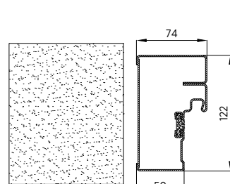
Rys. 10. Ościeżnica wewnętrzna z przekładką termiczną
