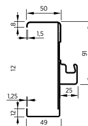
Rys. 57. Ościeżnica obejmująca
