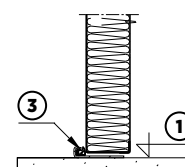
Rys. 88. Przekrój przez próg
