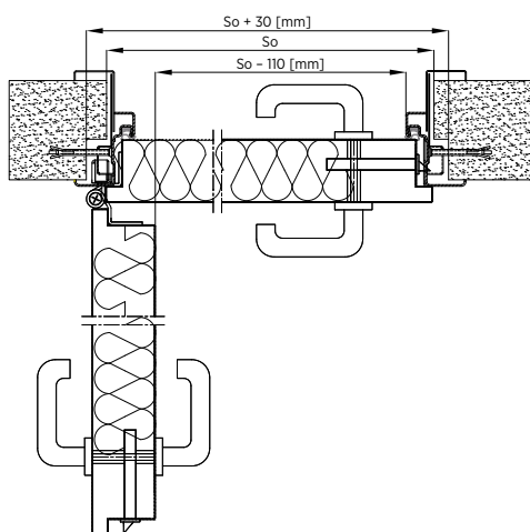
Rys. 48. Montaż do muru drzwi jednoskrzydłowych płaszczonek ECO TECH z ościeżnicą obejmującą bez przekładki termicznej – przekrój poziomy
