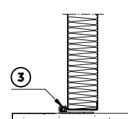
Rys. 64. Przekrój przez próg 3 - próg
