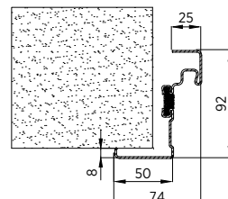
Rys. 9. Ościeżnica narożna z przekładką termiczną
