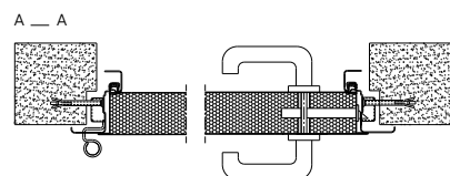
Rys. 3. Przekrój poziomy drzwi stalowych płaszczonek zewnętrznych ECO z ościeżnicą narożną bez przekładki termicznej
