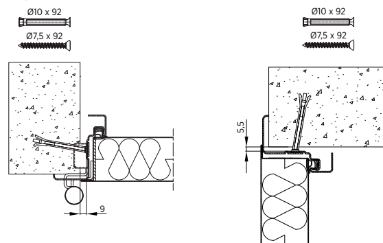
Rys. 33. Montaż ościeżnicy narożnej, boki i nadproże drzwi jednoskrzydłowych
