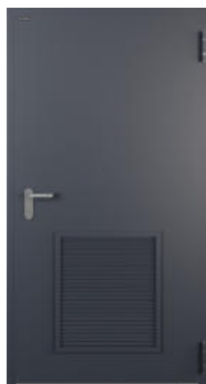
Rys. 44. Kratka wentylacyjna stalowa 525x625 [mm]
