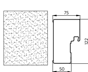
Rys. 7. Ościeżnica wewnętrzna
