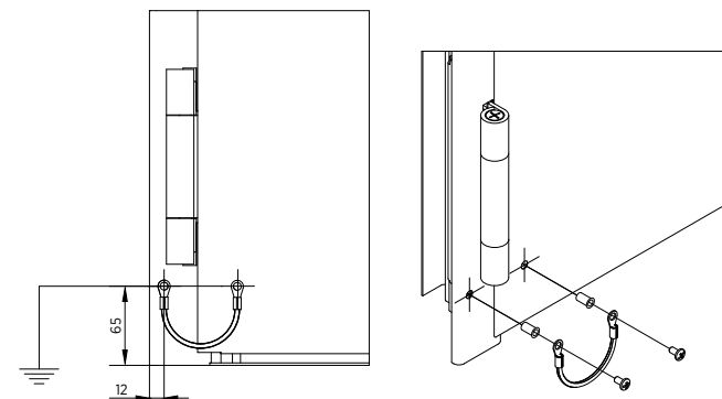
Rys. 33. Sposób wykonania uziemienia drzwi ECO
