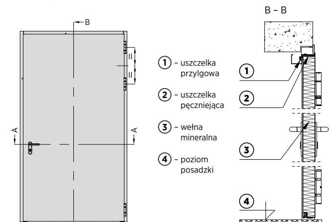
Rys. 1. Drzwi stalowe płaszczowe jednoskrzydłowe przeciwpożarowe EI120
