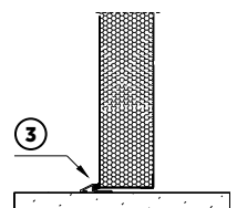
Rys. 31. Przekrój przez próg aluminiowy przykręcany
