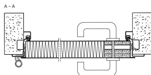
Rys. 74. Przekrój poziomy drzwi stalowych płaszczyse przeciwpożarowych wielkogabarytowych z ościeżnicą narożną
