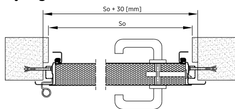
Rys. 50. Montaż do muru drzwi jednoskrzydłowych z ościeżnicą narożną bez przekładki termicznej – przekrój poziomy
