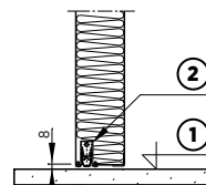
Rys. 87. Przekrój przez listwę opadającą
