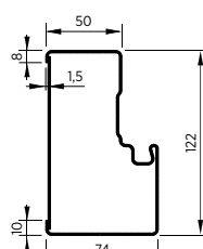
Rys. 56. Ościeżnica wewnętrzna
