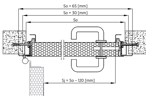
Rys. 58. Montaż do muru drzwi jednoskrzydłowych – ościeżnica narożna z przekładką termiczną – przekrój poziomy
