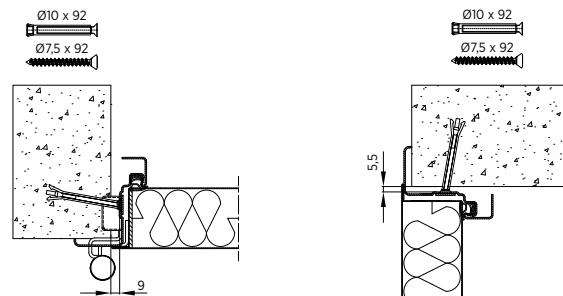
Rys. 70. Montaż ościeżnicy narożnej, boki i nadproże drzwi jednoskrzydłowych
