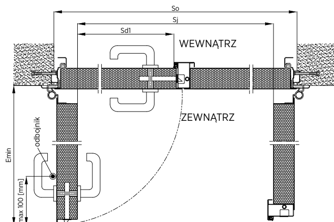
Rys. 71. Montaż przed otworem drzwi dwuskrzydłowych – ościeżnica narożna bez przekładki termicznej – przekrój poziomy
