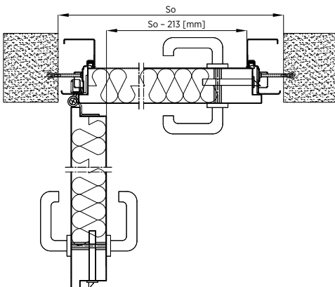
Rys. 50. Montaż do muru drzwi jednoskrzydłowych płaszczonek ECO TECH z ościeżnicą wewnętrzną bez przekładki termicznej – przekrój poziomy
