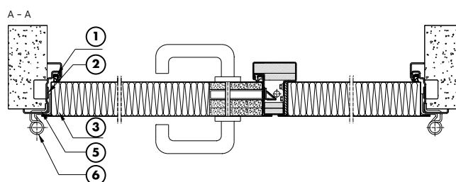
Rys. 52. Przekrój poziomy drzwi stalowych dwuskrzydłowych płaszczone przeciwpożarowych wielkogabarytowych z ościeżnicą narożną
