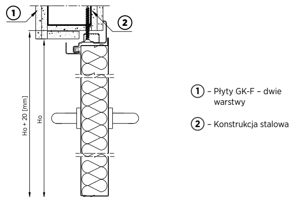
Rys. 43. Montaż do konstrukcji stalowej drzwi dwuskrzydłowych z ościeżnicą narożną - przekrój pionowy
