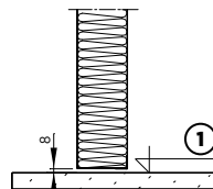
Rys. 62. Szczelina dolna drzwi bez progu 1 - poziom posadzki
