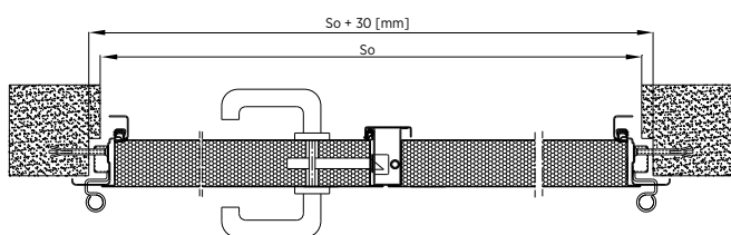
Rys. 52. Montaż do muru drzwi dwuskrzydłowych z ościeżnicą narożną bez przekładki termicznej – przekrój poziomy
