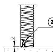
Rys. 63. Przekrój przez listwę opadającą 2 - listwa opadająca
