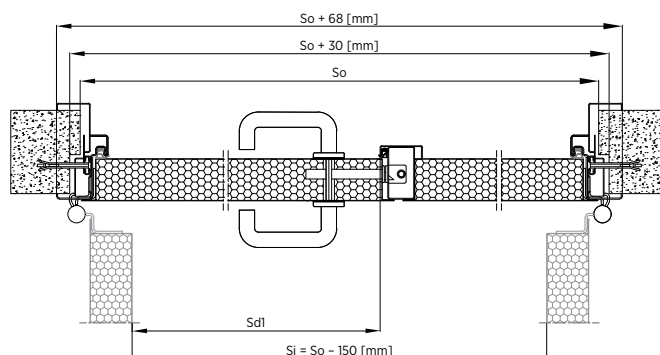
Rys. 64. Montaż do muru drzwi dwuskrzydłowych – ościeżnica obejmująca z przekładką termiczną – przekrój poziomy
