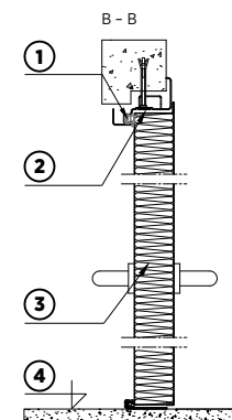
Rys. 40. Przekrój pionowy drzwi stalowych dwuskrzydłowych płaszczych przeciwpożarowych z ościeżnicą narożną
