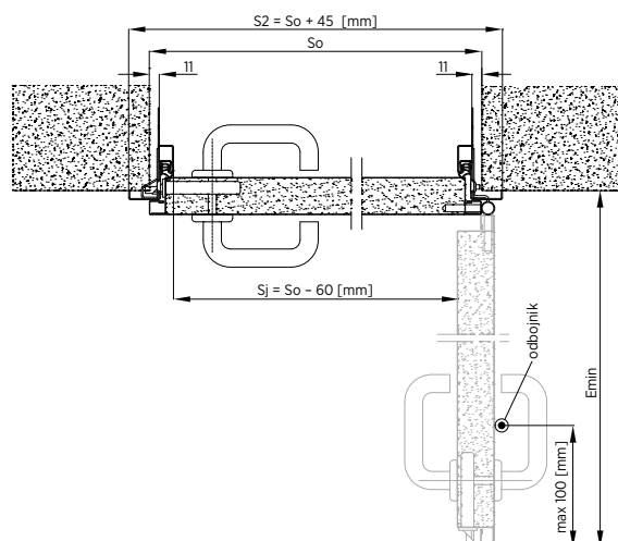
Rys. 28. Montaż drzwi jednoskrzydłowych z ościeżnicą narożną – przekrój poziomy
