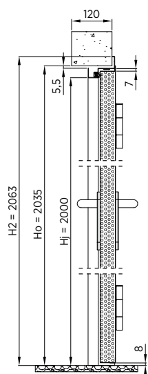
Rys. 19. Montaż do muru drzwi jednoskrzydłowych z ościeżnicą narożną - przekrój pionowy
