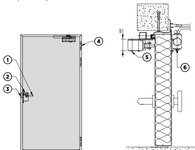
Rys. 72. Schemat drzwi jednoskrzydłowych – przekrój pionowy z układem napowietrzania
