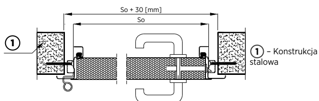
Rys. 54. Montaż do konstrukcji stalowej drzwi jednoskrzydłowych z ościeżnicą narożną bez przekładki termicznej – przekrój poziomy
