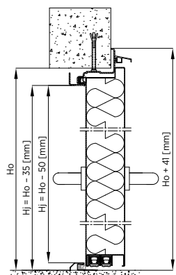
Rys. 47. Montaż do muru drzwi jednoskrzydłowych płaszczonek ECO TECH z ościeżnicą narożną bez przekładki termicznej – przekrój pionowy
