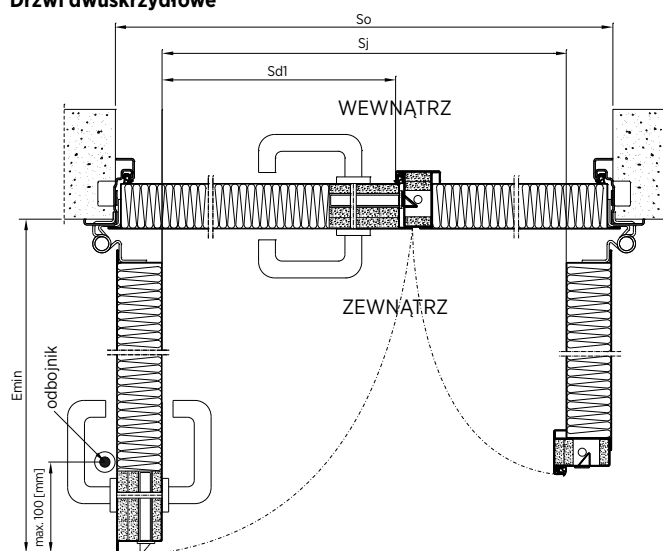
Rys. 46. Montaż na ościeżnicy narożnej drzwi dwuskrzydłowych – przekrój poziomy
