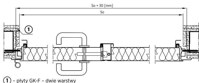
Rys. 42. Montaż do konstrukcji stalowej drzwi dwuskrzydłowych z ościeżnicą narożną - przekrój poziomy
