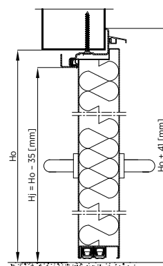
Rys. 53. Montaż do konstrukcji stalowej drzwi jednoskrzydłowych płaszczonek ECO TECH z ościeżnicą narożną bez przekładki termicznej – przekrój pionowy
