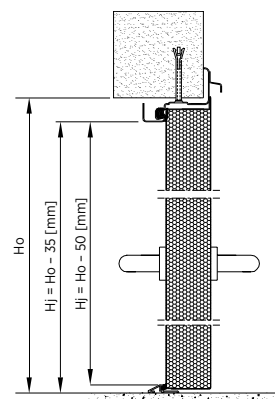
Rys. 51. Montaż do muru drzwi jednoskrzydłowych z ościeżnicą narożną bez przekładki termicznej – przekrój pionowy
