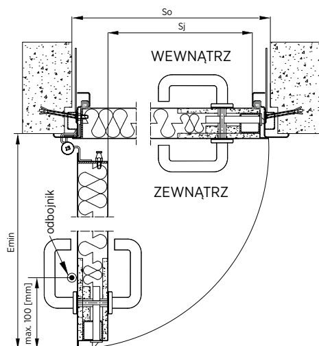
Rys. 77. Montaż na ościeżnicy narożnej – przekrój poziomy
