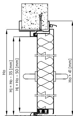
Rys. 49. Montaż do muru drzwi jednoskrzydłowych płaszczonek ECO TECH z ościeżnicą obejmującą bez przekładki termicznej – przekrój pionowy
