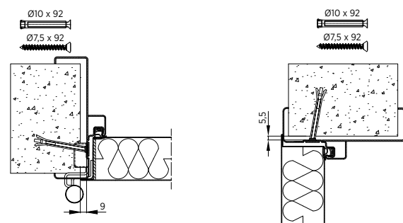
Rys. 71. Montaż ościeżnicy obejmującej, boki i nadproże drzwi jednoskrzydłowych
