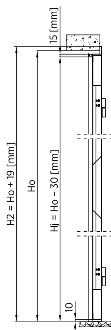
Rys. 10. Montaż do muru drzwi jednoskrzydłowych z ościeznicą narożną – przekrój pionowy
