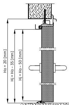
Rys. 57. Montaż do konstrukcji stalowej drzwi dwuskrzydłowych z ościeżnicą narożną bez przekładki termicznej – przekrój pionowy
