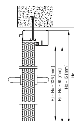
Rys. 67. Montaż do muru drzwi jednoskrzydłowych – ościeżnica wewnętrzna z przekładką termiczną – przekrój pionowy
