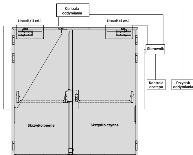
Rys. 75. Schemat podłączenia elementów układu napowietrzania drzwi stalowych płaszczone dwuskrzydłowych z funkcją paniczną
