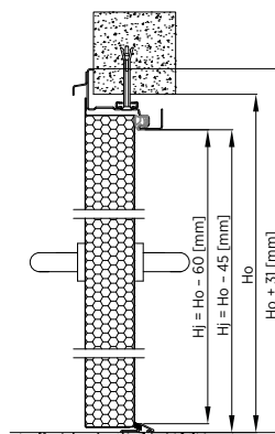
Rys. 59. Montaż do muru drzwi jednoskrzydłowych – ościeżnica narożna z przekładką termiczną – przekrój pionowy
