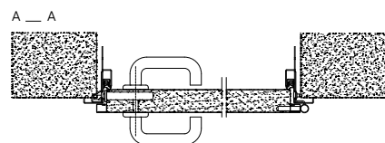
Rys. 3. Przekrój poziomy drzwi stalowych płaszczyznowych zewnętrznych do pomieszczeń nieogrzewanych ECO BASIC z ościeżnicą narożną
