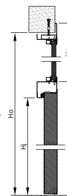
Rys. 87. Naświetle górne – przekrój pionowy
