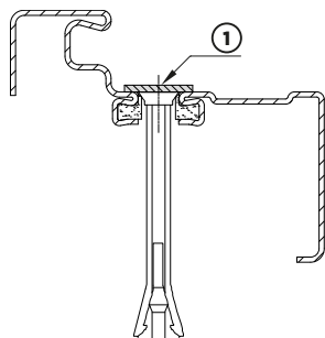
Rys. 89. Taśma maskująca otwory montażowe w ościeżnicy z przegrodą termiczną
