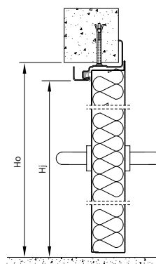
Rys. 45. Montaż na ościeżnicy narożnej - przekrój pionowy
