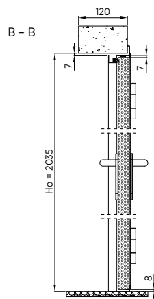
Rys. 2. Przekrój pionowy drzwi stalowych płaszczyznowych wewnętrznych DSp EI30 BASIC z ościeżnicą narożną
