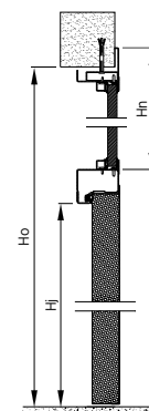
Rys. 84. Naświetle górne – przekrój pionowy
