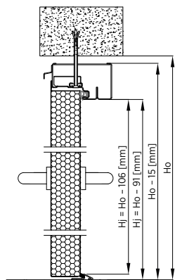
Rys. 69. Montaż do muru drzwi dwuskrzydłowych – ościeżnica wewnętrzna z przekładką termiczną – przekrój pionowy
