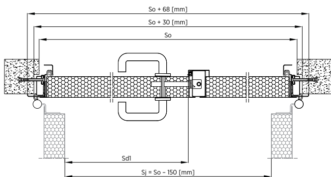
Rys. 60. Montaż do muru drzwi dwuskrzydłowych – ościeżnica narożna z przekładką termiczną – przekrój poziomy
