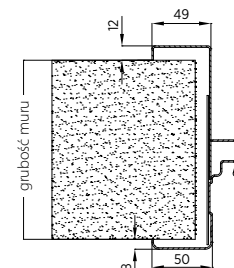
Rys. 8. Ościeżnica obejmująca
