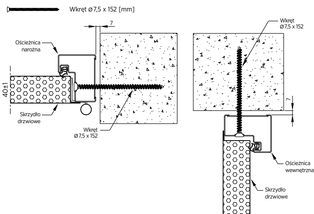
Rys. 17. Montaż ościeżnicy wewnętrznej z ościeżnicą wewnętrzną, boki i nadproże drzwi jednoskrzydłowych
