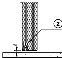
Rys. 30. Przekrój przez listwę opadającą
