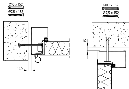
Rys. 35. Montaż ościeżnicy wewnętrznej, boki i nadproże drzwi jednoskrzydłowych
