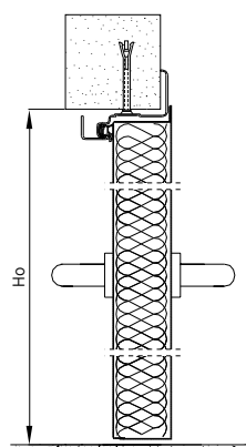
Rys. 37. Montaż do muru drzwi jednoskrzydłowych z ościeżnicą narożną – przekrój pionowy
