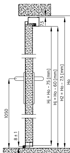
Rys. 31. Montaż do muru drzwi jednoskrzydłowych z ościeżnicą wewnętrzną – przekrój pionowy
