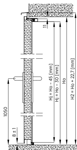
Rys. 29. Montaż do muru drzwi jednoskrzydłowych z ościeżnicą narożną – przekrój pionowy
