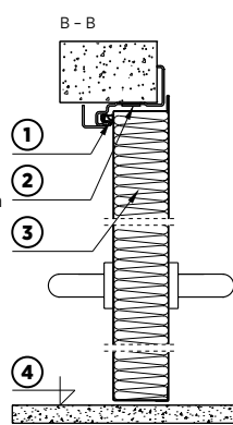
Rys. 73. Przekrój pionowy drzwi stalowych płaszczyse przeciwpożarowych z ościeżnicą narożną
