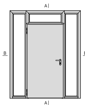
Rys. 83. Drzwi jednoskrzydłowe ECO z doświetlami bocznymi i naświetlem górnym
