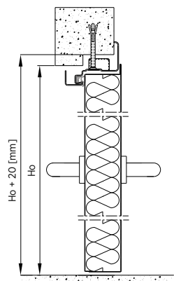
Rys. 39. Montaż do muru drzwi dwuskrzydłowych z ościeżnicą narożną - przekrój pionowy
