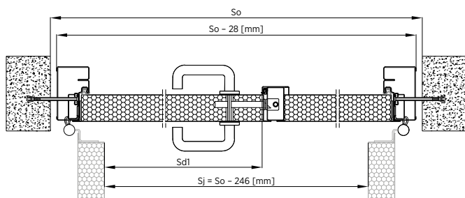
Rys. 68. Montaż do muru drzwi dwuskrzydłowych – ościeżnica wewnętrzna z przekładką termiczną – przekrój poziomy
