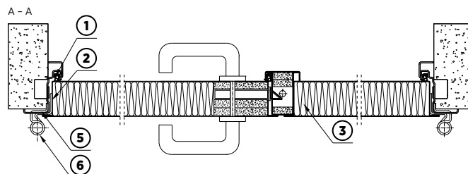
Rys. 41. Przekrój poziomy drzwi stalowych dwuskrzydłowych płaszczych przeciwpożarowych z ościeżnicą narożną
