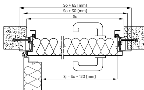
Rys. 54. Montaż do muru drzwi jednoskrzydłowych – ościeżnica narożna z przekładką termiczną – przekrój poziomy
