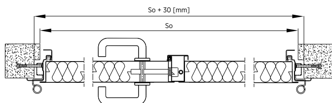
Rys. 38. Montaż do muru drzwi dwuskrzydłowych z ościeżnicą narożną - przekrój poziomy
