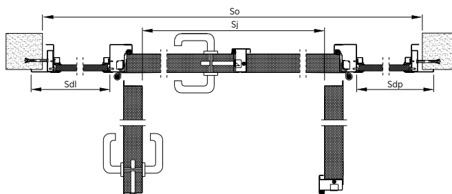
Rys. 88. Doświetla boczne – przekrój poziomy
