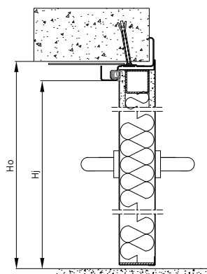
Rys. 78. Montaż na ościeżnicy narożnej – przekrój pionowy
