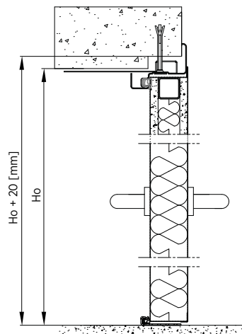
Rys. 99. Montaż do muru drzwi dwuskrzydłowych z ościeżnicą narożną – przekrój pionowy
