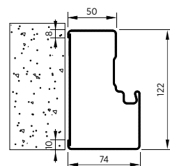
Rys. 10. Ościeżnica wewnętrzna
