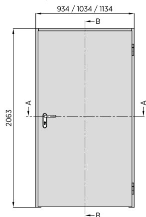
Rys. 1. Drzwi stalowe płaszczowe DSp EI30 BASIC jednoskrzydłowe
