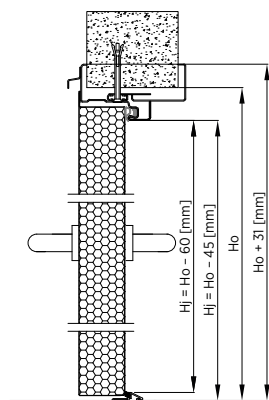
Rys. 63. Montaż do muru drzwi jednoskrzydłowych – ościeżnica obejmująca z przekładką termiczną – przekrój pionowy
