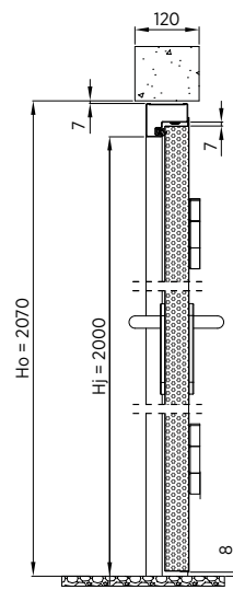
Rys. 21. Montaż do muru drzwi jednoskrzydłowych z ościeżnicą wewnętrzną - przekrój pionowy
