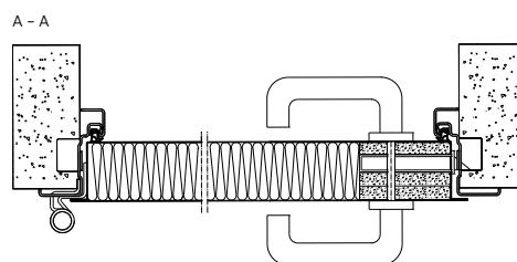
Rys. 38. Przekrój poziomy drzwi stalowych płaszczych przeciwpożarowych z ościeżnicą narożną
