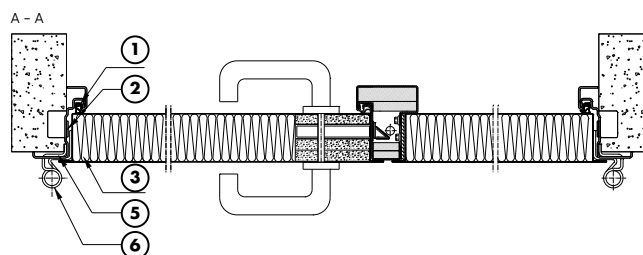
Rys. 77. Przekrój poziomy drzwi stalowych dwuskrzydłowych płaszczyse przeciwpożarowych wielkogabarytowych z ościeżnicą narożną
