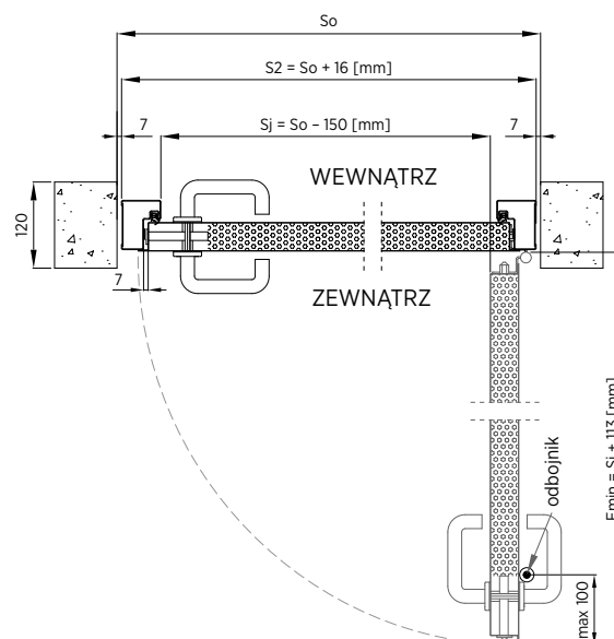
Rys. 20. Montaż drzwi jednoskrzydłowych z ościeżnicą wewnętrzną - przekrój poziomy
