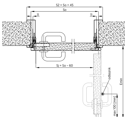
Rys. 32. Montaż drzwi jednoskrzydłowych z ościeżnicą obejmującą – przekrój poziomy
