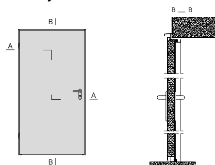
Rys. 1. Drzwi stalowe płaszczyznowe ECO BASIC
