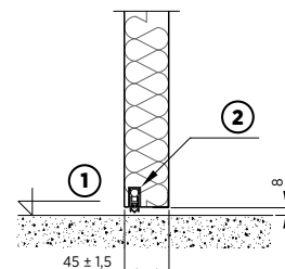
Rys. 15. Przekrój przez listwę opadającą
