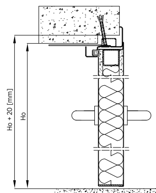
Rys. 76. Montaż do muru drzwi dwuskrzydłowych z ościeżnicą narożną – przekrój pionowy
