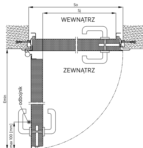
Rys. 70. Montaż przed otworem – ościeżnica narożna bez przekładki termicznej – przekrój poziomy
