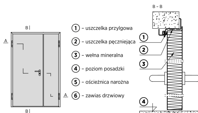
Rys. 50. Drzwi stalowe dwuskrzydłowe płaszczone przeciwpożarowe wielkogabarytowe
