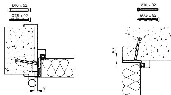
Rys. 94. Montaż ościeżnicy obejmującej, boki i nadproże drzwi jednoskrzydłowych
