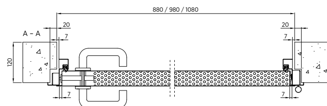
Rys. 3. Przekrój poziomy drzwi stalowych płaszczykowych wewnętrznych DSp EI30 BASIC z ościeżnicą narożną
