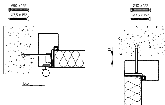
Rys. 72. Montaż ościeżnicy wewnętrznej, boki i nadproże drzwi jednoskrzydłowych
