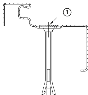
Rys. 90. Taśma maskująca otwory montażowe w ościeżnicy bez przegrody termicznej
