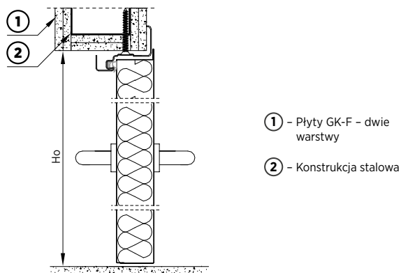
Rys. 41. Montaż do konstrukcji stalowej drzwi jednoskrzydłowych z ościeżnicą narożną - przekrój pionowy
