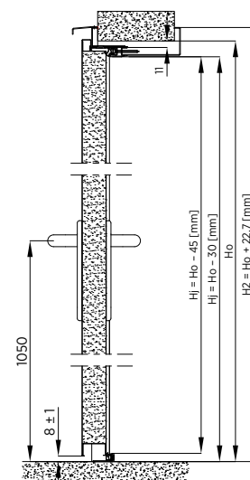
Rys. 33. Montaż do muru drzwi jednoskrzydłowych z ościeżnicą obejmującą – przekrój pionowy
