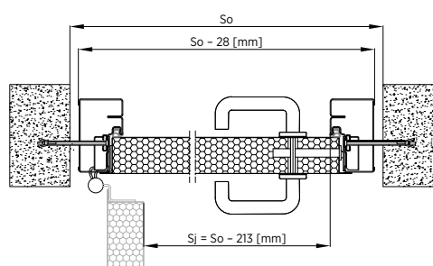
Rys. 66. Montaż do muru drzwi jednoskrzydłowych – ościeżnica wewnętrzna z przekładką termiczną – przekrój poziomy
