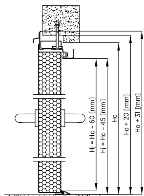
Rys. 61. Montaż do muru drzwi dwuskrzydłowych – ościeżnica narożna z przekładką termiczną – przekrój pionowy
