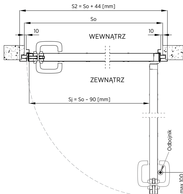
Rys. 9. Montaż drzwi UTILITY jednoskrzydłowych z ościeznicą narożną – przekrój poziomy
