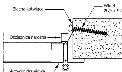
Rys. 8. Montaż ościeznicy narożnej, bok drzwi jednoskrzydłowych
