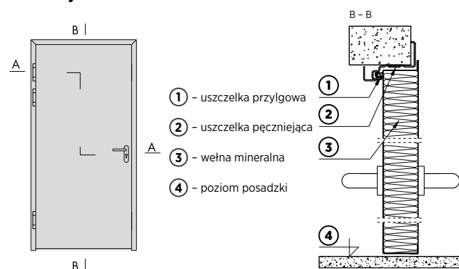
Rys. 47. Drzwi stalowe płaszczone jednoskrzydłowe przeciwpożarowe
