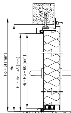
Rys. 55. Montaż do muru drzwi jednoskrzydłowych – ościeżnica narożna z przekładką termiczną – przekrój pionowy
