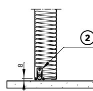
Rys. 27. Przekrój przez listwę opadającą
