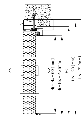
Rys. 65. Montaż do muru drzwi dwuskrzydłowych – ościeżnica obejmująca z przekładką termiczną – przekrój pionowy
