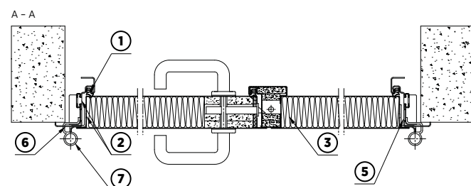
Rys. 6. Przekrój poziomy drzwi stalowych płaszczone dwuskrzydłowych przeciwpożarowych z przekładką termiczną
