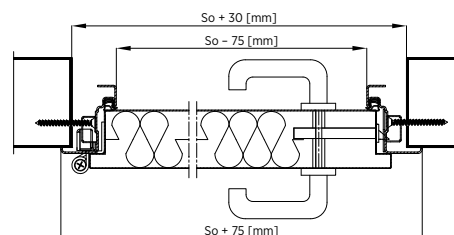
Rys. 52. Montaż do konstrukcji stalowej drzwi jednoskrzydłowych płaszczonek ECO TECH z ościeżnicą narożną bez przekładki termicznej – przekrój poziomy
