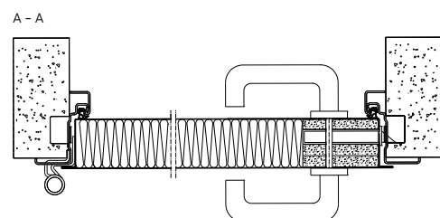
Rys. 49. Przekrój poziomy drzwi stalowych płaszczone przeciwpożarowych wielkogabarytowych z ościeżnicą narożną
