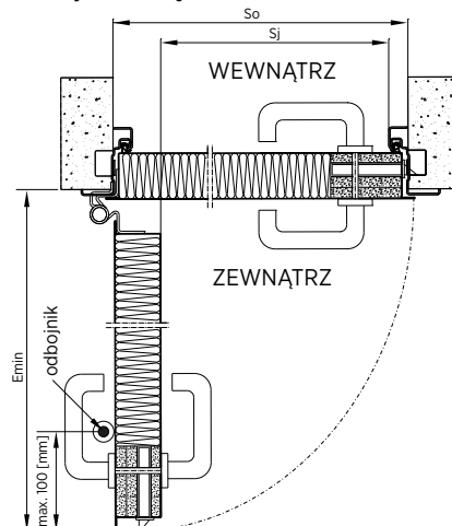
Rys. 44. Montaż na ościeżnicy narożnej - przekrój poziomy
