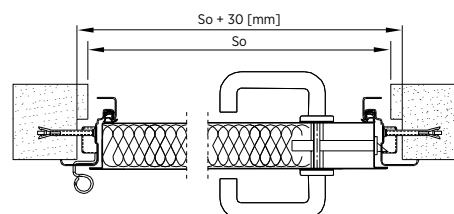
Rys. 36. Montaż do muru drzwi jednoskrzydłowych z ościeżnicą narożną – przekrój poziomy
