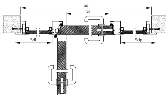
Rys. 85. Doświetla boczne – przekrój poziomy
