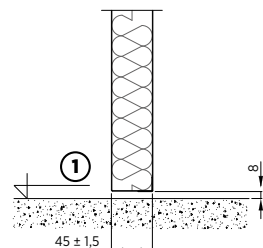
Rys. 14. Szczelina dolna drzwi bez progu
