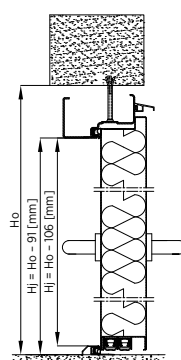
Rys. 51. Montaż do muru drzwi jednoskrzydłowych płaszczonek ECO TECH z ościeżnicą wewnętrzną bez przekładki termicznej – przekrój pionowy
