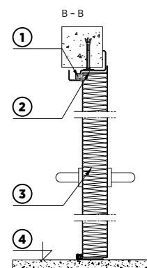
Rys. 37. Przekrój pionowy drzwi stalowych płaszczych przeciwpożarowych z ościeżnicą narożną
