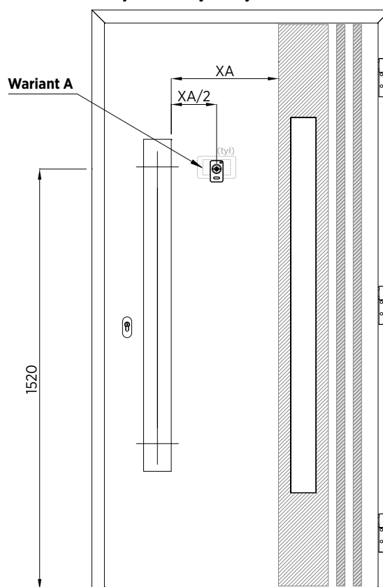
Rys. 68. Wizjer od strony uchwytu – przykład montażu dla wzoru 004
