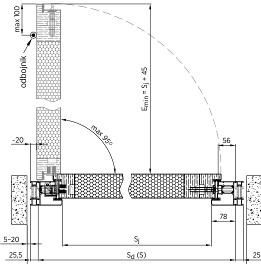
Rys. 74. Montaż w otworze – przekrój poziomy – drzwi NOVA z zawiasami ukrytymi i poszerzenia z obu stron – drzwi otwierane do wewnątrz
