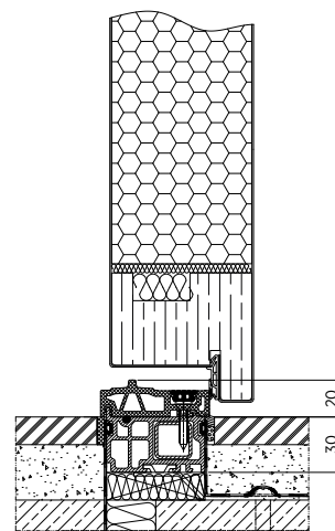
Rys. 55. Montaż progu z zastosowaniem profilu podprogowego o wysokości 30 [mm]
