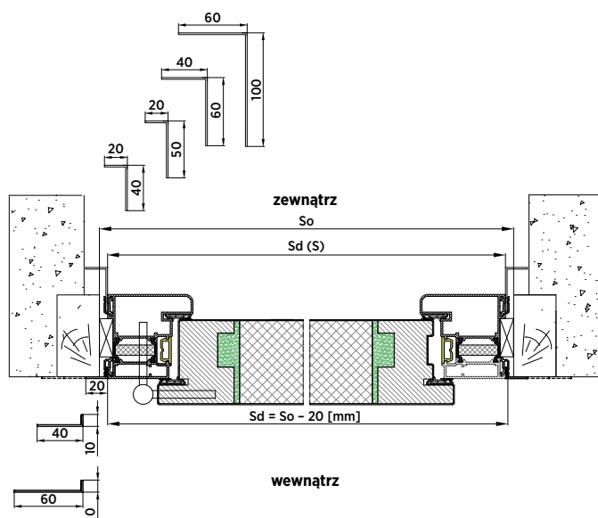
Rys. 90. Montaż w otworze z kątownikiem renowacyjnym od wewnątrz i od zewnątrz – przekrój poziomy – drzwi NOVA
