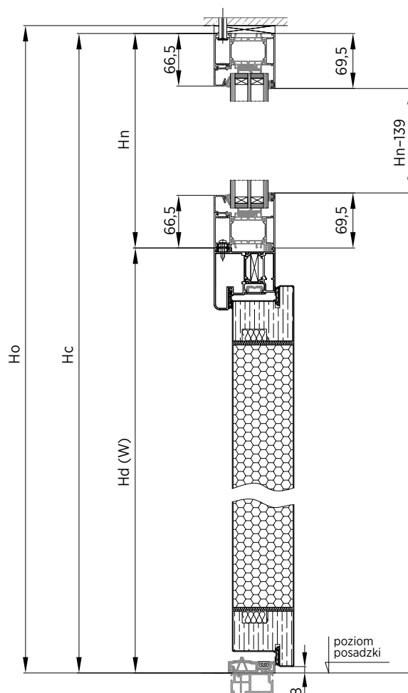
Rys. 97. Zależności wymiarowe dla naświetla górnego
