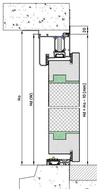
Rys. 87. Montaż w otworze z kątownikiem renowacyjnym od wewnątrz i od zewnątrz – przekrój pionowy – drzwi NOVA
