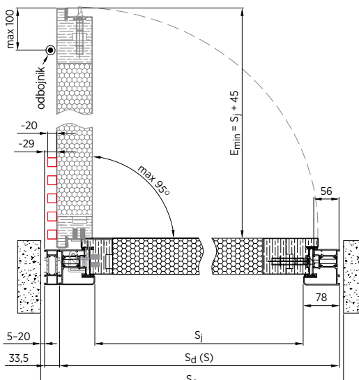
Rys. 78. Montaż w otworze – przekrój poziomy – drzwi NOVA z zawiasami ukrytymi i poszerzenia z obu stron – drzwi otwierane do wewnątrz
