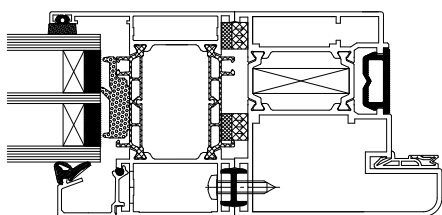
Rys. 83. Połączenie ościeżnicy z doświetlem / naświetlem (kierunek otwierania drzwi - na zewnątrz)
