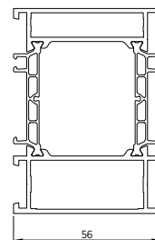
Rys. 94. Poszerzenie – szer. 56 [mm]
