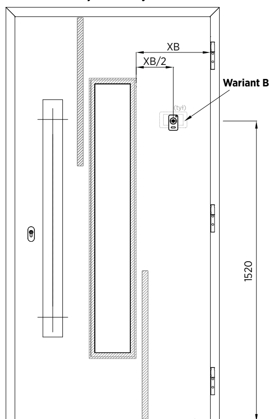
Rys. 69. Wizjer od strony zawiasów – przykład montażu dla wzoru 002
