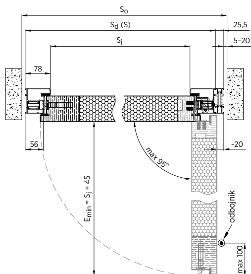
Rys. 71. Montaż w otworze – przekrój poziomy – drzwi NOVA z zawiasami ukrytymi i poszerzeniem z jednej strony – drzwi otwierane na zewnątrz
