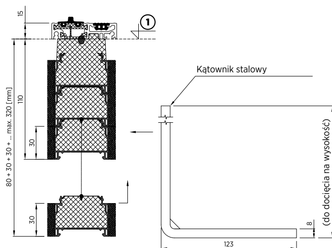
Rys. 61. Próg aluminiowy
