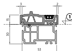
Rys. 53. Próg tworzywowy z zamontowanym profilem tworzywowym podprogowym
