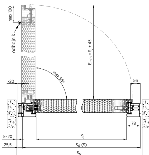
Rys. 72. Montaż w otworze – przekrój poziomy – drzwi NOVA z zawiasami ukrytymi i poszerzeniem z jednej strony – drzwi otwierane do wewnątrz
