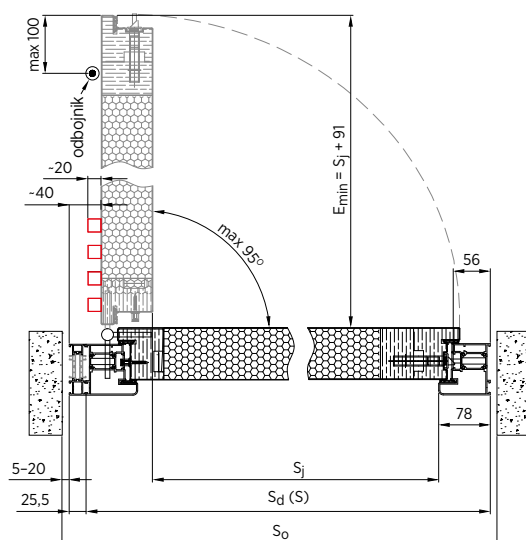
Rys. 76. Montaż w otworze – przekrój poziomy – drzwi NOVA z zawiasami 3D i poszerzeniem z jednej strony – drzwi otwierane do wewnątrz
