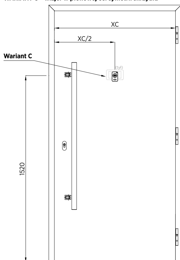
Rys. 70. Wizjer w pionowej osi symetrii skrzydła – przykład montażu dla wzoru 001
