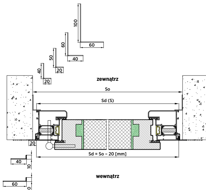
Rys. 88. Montaż w otworze z kątownikiem renowacyjnym od wewnątrz i od zewnątrz – przekrój poziomy – drzwi NOVA
