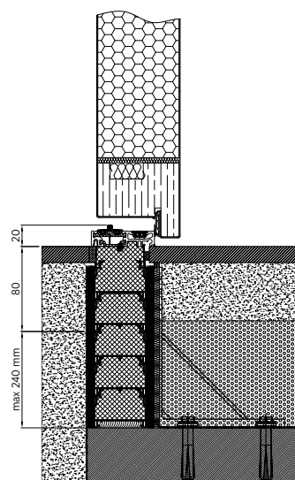
Rys. 60. Możliwość zastosowania dodatkowych profili o wysokości 30 [mm]. Maksymalna wysokość całego termo-poszerzenia to 320 [mm]. Powyżej wysokości 90 [mm] dodatkowego termo-poszerzenia należy go zamontować na kątownikach mocujących
