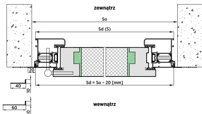
Rys. 86. Montaż w otworze z kątownikiem renowacyjnym od wewnątrz – przekrój poziomy – drzwi NOVA
