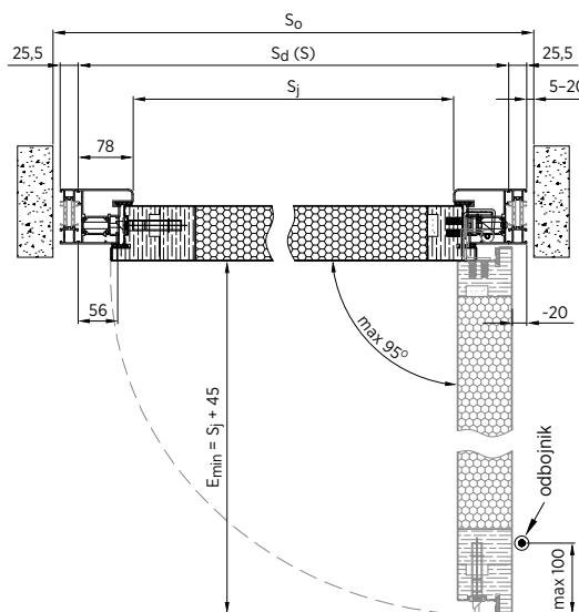
Rys. 73. Montaż w otworze – przekrój poziomy – drzwi NOVA z zawiasami ukrytymi i poszerzenia z obu stron – drzwi otwierane na zewnątrz
