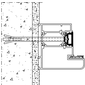
Rys. 80. Montaż bezpośredni za pomocą kołków rozporowych przez ościeżnicę (brak otworowania pod kołki w profilu)
