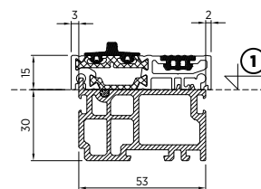
Rys. 54. Próg aluminiowy z zamontowanym profilem tworzywowym podprogowym
