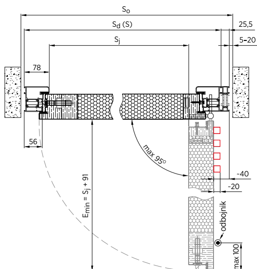
Rys. 75. Montaż w otworze – przekrój poziomy – drzwi NOVA z zawiasami 3D i poszerzeniem z jednej strony – drzwi otwierane na zewnątrz
