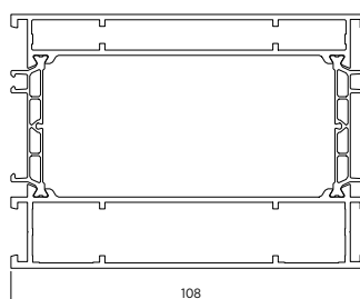
Rys. 95. Poszerzenie – szer. 108 [mm]
