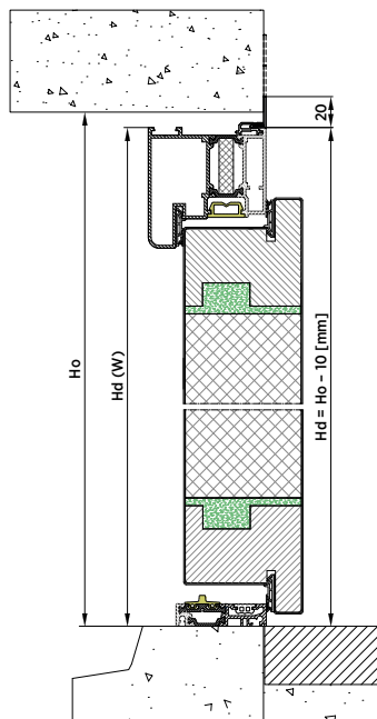
Rys. 85. Montaż w otworze z kątownikiem renowacyjnym od wewnątrz – przekrój pionowy – drzwi NOVA
