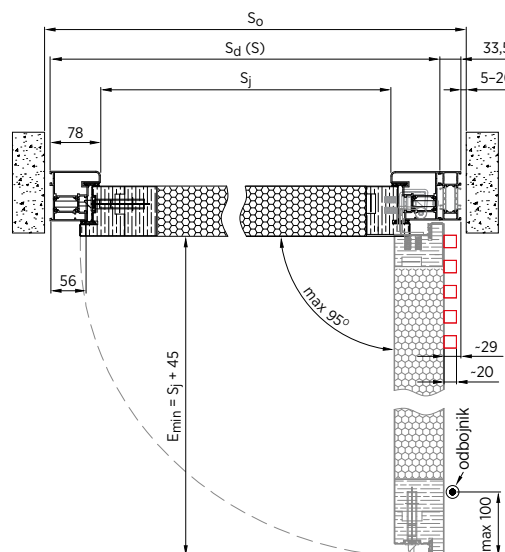
Rys. 77. Montaż w otworze – przekrój poziomy – drzwi NOVA z zawiasami ukrytymi i poszerzenia z obu stron – drzwi otwierane na zewnątrz
