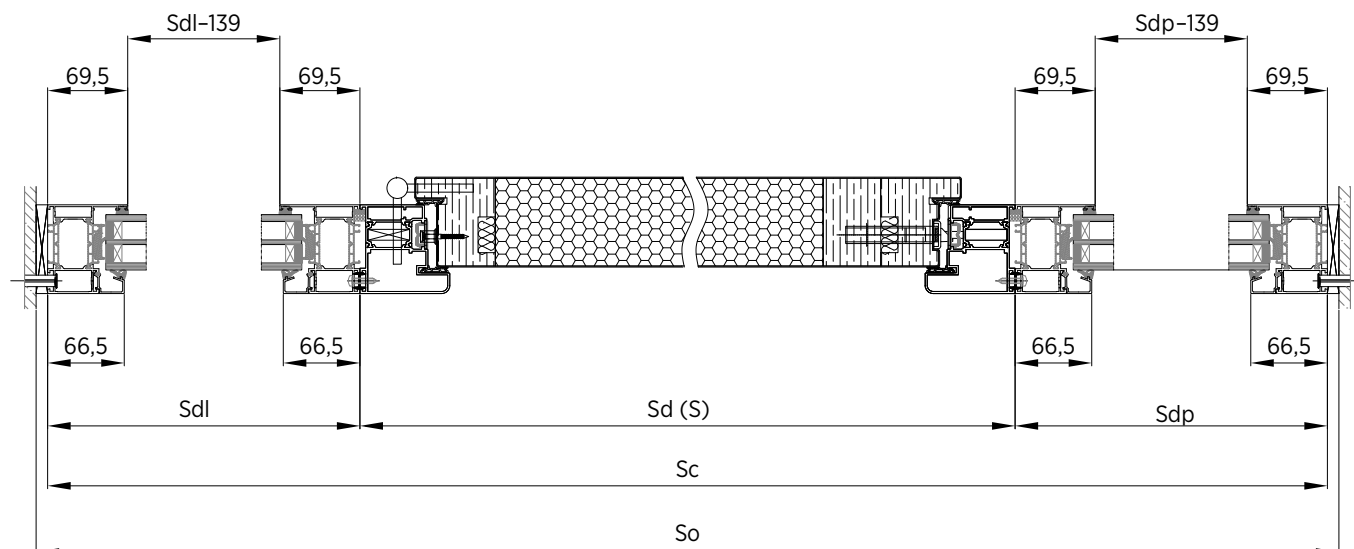
Rys. 96. Zależności wymiarowe dla doświetli bocznych
