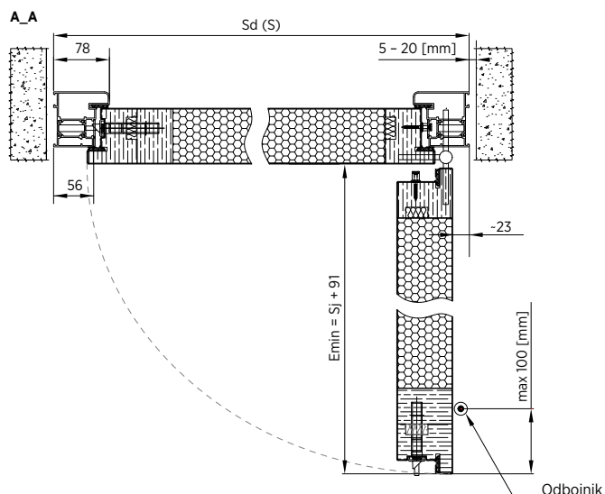
Rys. 4. Przekrój poziomy drzwi NOVA
