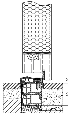
Rys. 56. Montaż progu z zastosowaniem dodatkowego profilu o wysokości 30 [mm] (maksymalna wysokość poszerzenia tego rozwiązania to 60 [mm])
