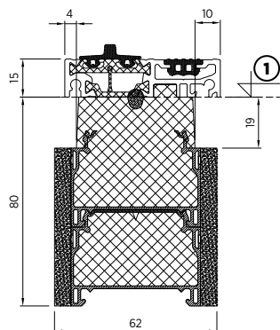
Rys. 57. Próg aluminiowy z zamontowanym termo-poszerzeniem Stropex 80 [mm]
