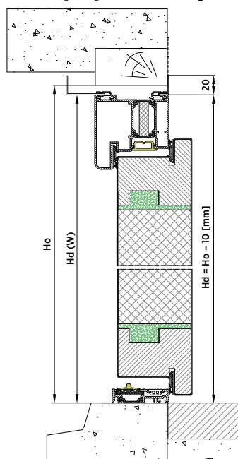
Rys. 89. Montaż w otworze z kątownikiem renowacyjnym od wewnątrz i od zewnątrz – przekrój pionowy – drzwi NOVA
