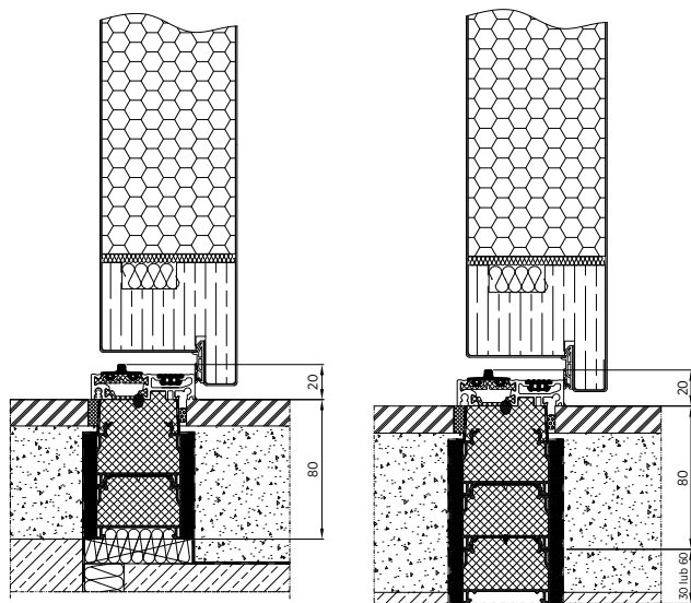
Rys. 58. Montaż progu z termo-poszerzeniem Stropex o wysokości 80 [mm]
