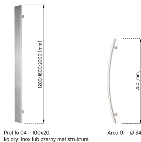
Rys. 33. Wzory uchwytów
