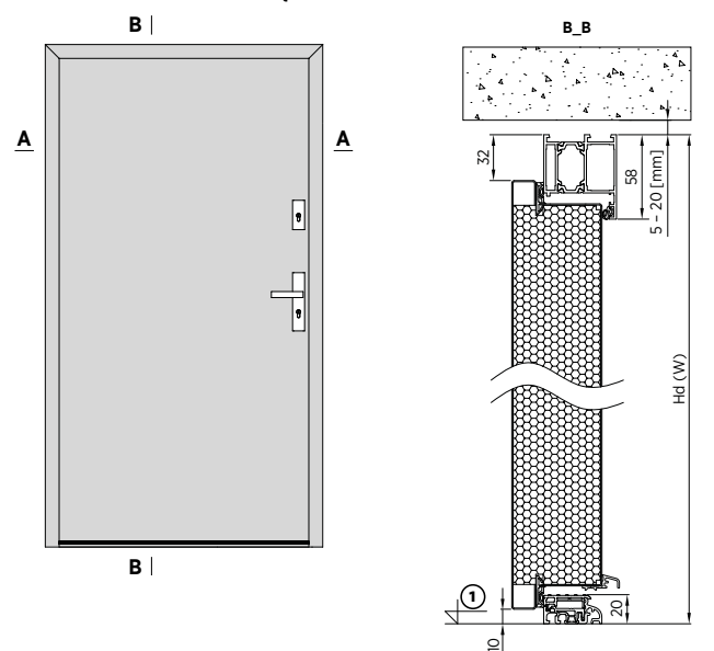
Rys. 6. Przekrój pionowy drzwi NOBE z ościeżnicą aluminiową – otwierane do wewnątrz
