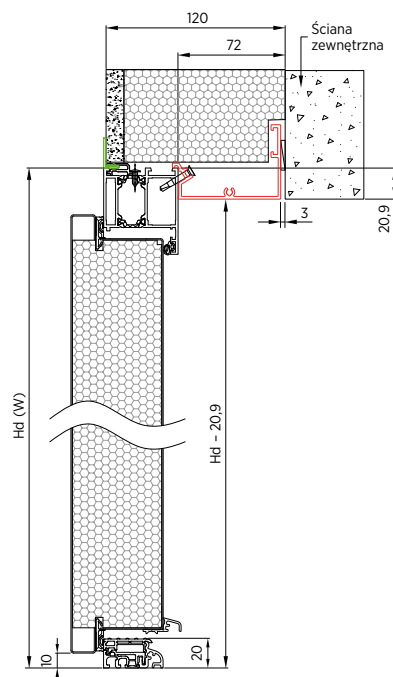
Rys. 40. Renowacja ISO 120 – przekrój pionowy – otwierane do wewnątrz – Drzwi NOBE
