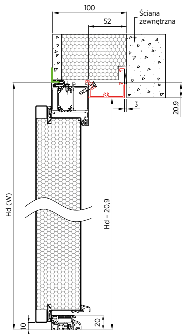
Rys. 38. Renowacja ISO 100 – przekrój pionowy – otwierane do wewnątrz – Drzwi NOBE
