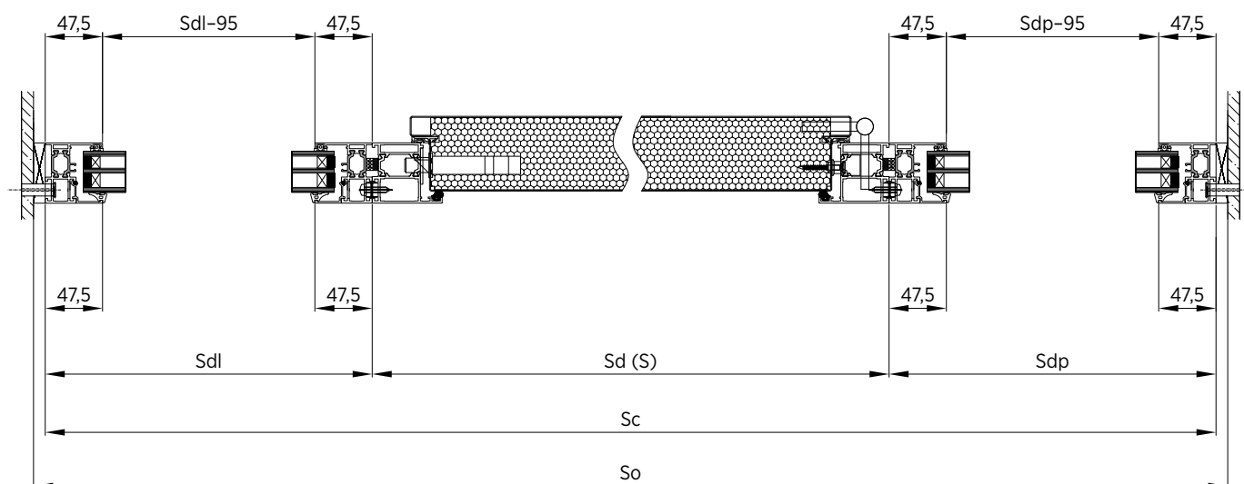
Rys. 53. Zależności wymiarowe dla doświetli bocznych
