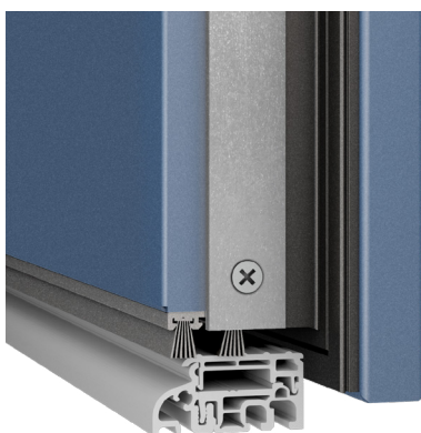
Rys. 34. Próg aluminiowo-tworzywowi 40 [mm] z dodatkowym doszczelnieniem progowym – drzwi otwierane na zewnątrz – rozwiązanie opcjonalne
