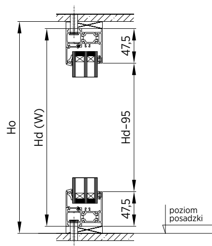
Rys. 54. Przekrój pionowy doświetla NOBE z ościeżnicą aluminiową
