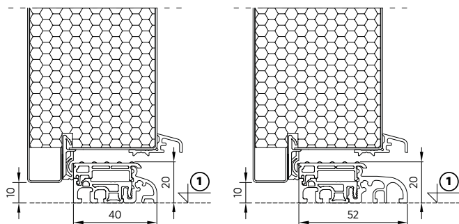
Rys. 32. Przekrój progu aluminiowo-tworzywowego 40 [mm] drzwi otwieranych do wewnątrz – rozwiązanie standardowe
