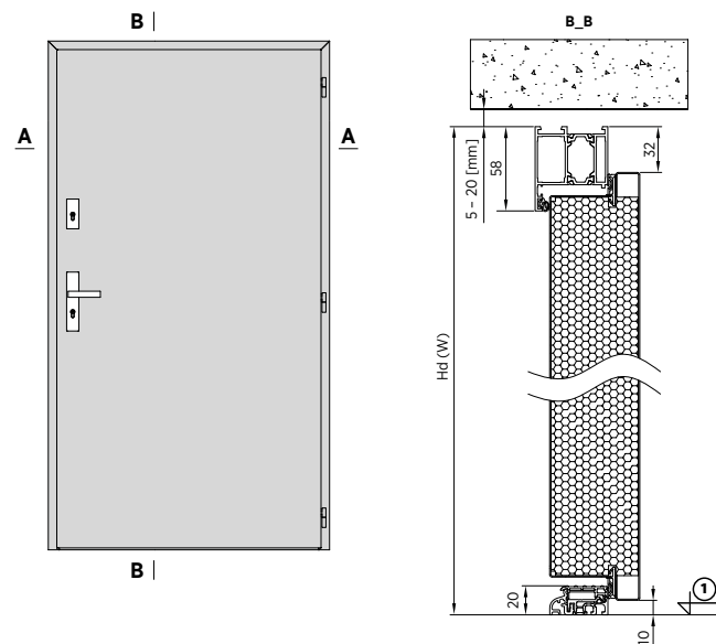
Rys. 3. Przekrój pionowy drzwi NOBE z ościeżnicą aluminiową – otwierane na zewnątrz
