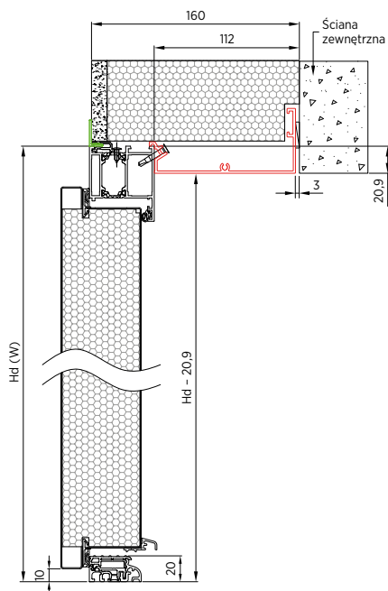
Rys. 42. Renowacja ISO 160 – przekrój pionowy – otwierane do wewnątrz – Drzwi NOBE
