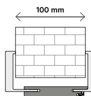
ZAKRES STANDARDOWY regulacja bez skróconego pióra kątownika
