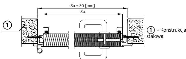
Rys. 51. Montaż do konstrukcji stalowej drzwi jednoskrzydłowych z ościeżnicą narożną bez przekładki termicznej – przekrój poziomy
