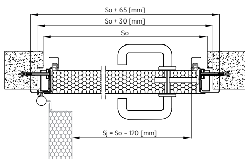
Rys. 55. Montaż do muru drzwi jednoskrzydłowych – ościeżnica narożna z przekładką termiczną – przekrój poziomy
