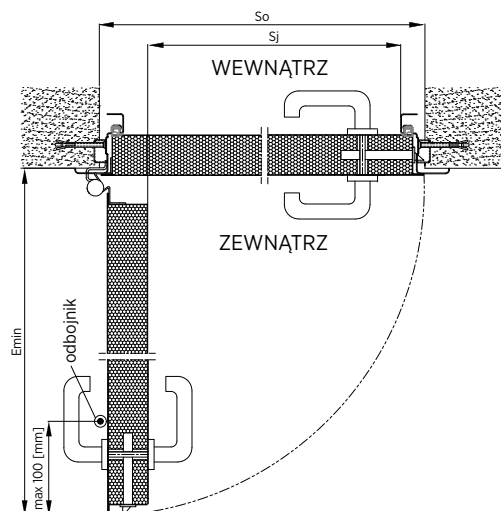
Rys. 67. Montaż przed otworem – ościeżnica narożna bez przekładki termicznej – przekrój poziomy
