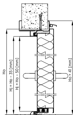
Rys. 49. Montaż do muru drzwi jednostronnych płaszczowych ECO TECH z ościeżnicą obejmującą bez przelączki termicznej – przekrój pionowy
