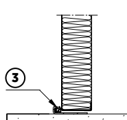
Rys. 26. Przekrój przez próg
