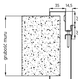
Rys. 8. Ościeżnica obejmująca (zakres regulacji ± 5 [mm])
