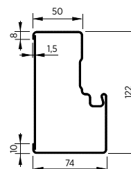
Rys. 10. Ościeżnica wewnętrzna
