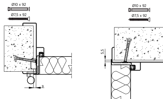
Rys. 32. Montaż ościeżnicy obejmującej, boki i nadproże drzwi jednoskrzydłowych
