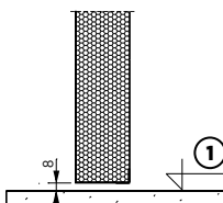
Rys. 27. Szczelina dolna drzwi bez progu
