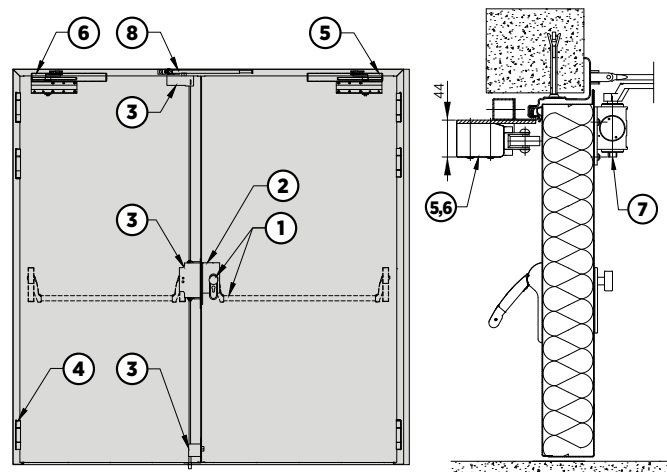
Rys. 71. Schemat układu napowietrzania drzwi stalowych płaszczone dwuskrzydłowych z funkcją paniczną – przekrój pionowy
