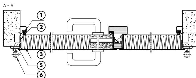
Rys. 77. Przekrój poziomy drzwi stalowych dwuskrzydłowych płaszczyne przeciwpożarowych wielkogabarytowych z ościeżnicą narożną
