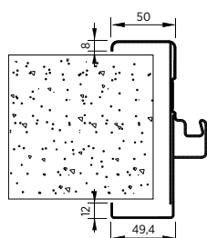
Rys. 11. Ościeżnica obejmująca
