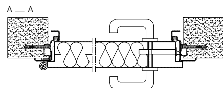
Rys. 3. Przekrój poziomy drzwi stalowych płaszczonek zewnętrznych ECO TECH z ościeżnicą narożną
