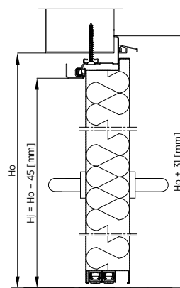
Rys. 63. Montaż do konstrukcji stalowej drzwi jednoskrzydłowych z ościeżnicą narożną z przekładką - przekrój pionowy
