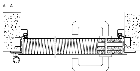
Rys. 38. Przekrój poziomy drzwi stalowych płaszczykowych przeciwpożarowych z ościeżnicą narożną
