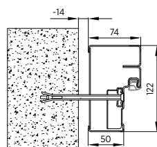
Rys. 13. Ościeżnica wewnętrzna z przekładką termiczną
