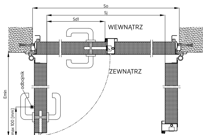
Rys. 68. Montaż przed otworem drzwi dwuskrzydłowych – ościeżnica narożna bez przekładki termicznej – przekrój poziomy
