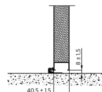
Rys. 20. Przekrój przez próg
