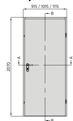
Rys. 1. Drzwi stalowe płaszczone ECO BASIC UNI
