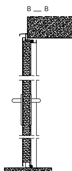
Rys. 2. Przekrój pionowy drzwi stalowych płaszczonek zewnętrznych do pomieszczeń nieogrzewanych ECO BASIC z ościeżnicą narożną
