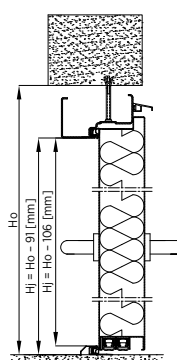
Rys. 51. Montaż do muru drzwi jednostronnych płaszczowych ECO TECH z ościeżnicą wewnętrzną bez przelączki termicznej – przekrój pionowy
