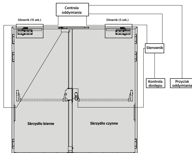
Rys. 72. Schemat podłączenia elementów układu napowietrzania drzwi stalowych płaszczone dwuskrzydłowych z funkcją paniczną
