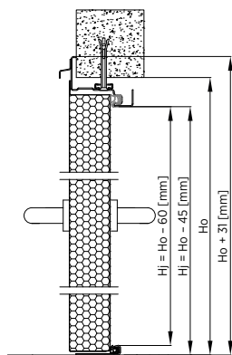
Rys. 56. Montaż do muru drzwi jednoskrzydłowych – ościeżnica narożna z przekładką termiczną – przekrój pionowy
