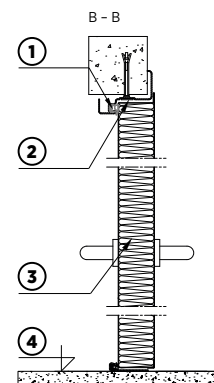
Rys. 37. Przekrój pionowy drzwi stalowych płaszczykowych przeciwpożarowych z ościeżnicą narożną
