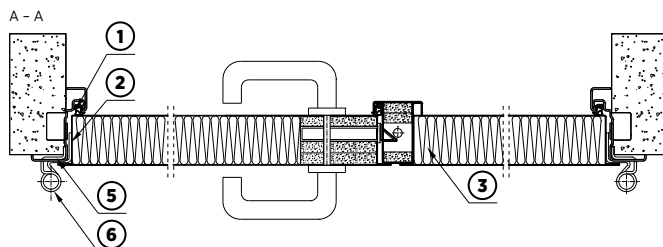
Rys. 41. Przekrój poziomy drzwi stalowych dwuskrzydłowych płaszczykowych przeciwpożarowych z ościeżnicą narożną
