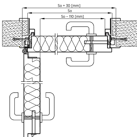
Rys. 48. Montaż do muru drzwi jednostronnych płaszczowych ECO TECH z ościeżnicą obejmującą bez przelączki termicznej – przekrój poziomy
