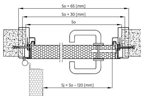
Rys. 59. Montaż do muru drzwi jednoskrzydłowych – ościeżnica obejmująca z przekładką termiczną – przekrój poziomy
