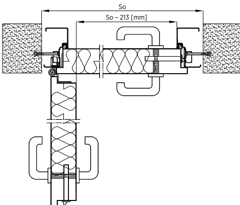
Rys. 50. Montaż do muru drzwi jednostronnych płaszczowych ECO TECH z ościeżnicą wewnętrzną bez przelączki termicznej – przekrój poziomy
