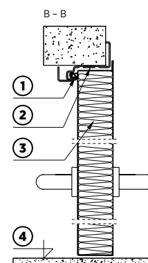
Rys. 5. Przekrój pionowy drzwi stalowych dwuskrzydłowych płaszczowych przeciwpożarowych z ościeżnicą narożną
