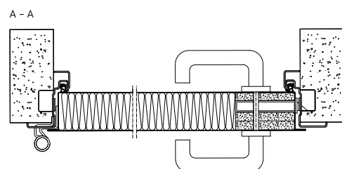
Rys. 74. Przekrój poziomy drzwi stalowych płaszczyne przeciwpożarowych wielkogabarytowych z ościeżnicą narożną
