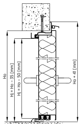
Rys. 47. Montaż do muru drzwi jednostronnych płaszczowych ECO TECH z ościeżnicą narożną bez przelączki termicznej – przekrój pionowy
