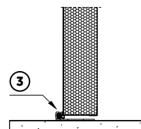
Rys. 29. Przekrój przez próg
