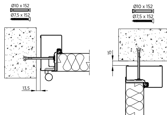
Rys. 33. Montaż ościeżnicy wewnętrznej, boki i nadproże drzwi jednoskrzydłowych
