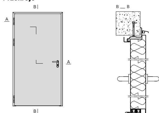
Rys. 1. Drzwi stalowe płaszczone ECO TECH jednoskrzydłowe
