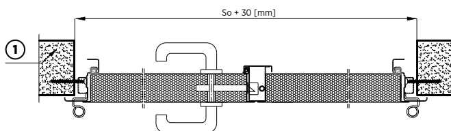
Rys. 53. Montaż do konstrukcji stalowej drzwi dwuskrzydłowych z ościeżnicą narożną bez przekładki termicznej – przekrój poziomy
