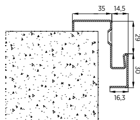
Rys. 6. Ościeżnica narożna
