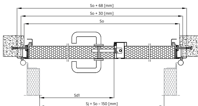
Rys. 57. Montaż do muru drzwi dwuskrzydłowych – ościeżnica narożna z przekładką termiczną – przekrój poziomy
