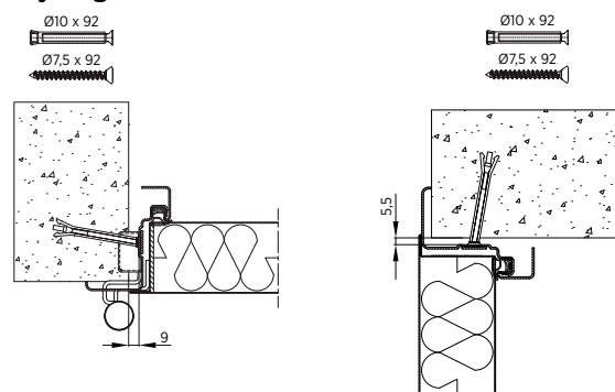
Rys. 31. Montaż ościeżnicy narożnej, boki i nadproże drzwi jednoskrzydłowych
