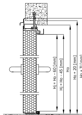
Rys. 58. Montaż do muru drzwi dwuskrzydłowych – ościeżnica narożna z przekładką termiczną – przekrój pionowy
