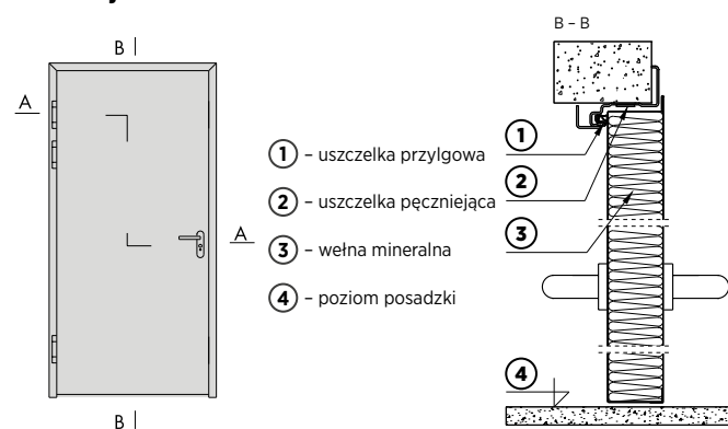
Rys. 72. Drzwi stalowe płaszczyne jednoskrzydłowe przeciwpożarowe
