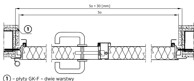
Rys. 40. Montaż do konstrukcji stalowej drzwi dwuskrzydłowych z ościeżnicą narożną – przekrój poziomy
