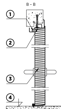
Rys. 40. Przekrój pionowy drzwi stalowych dwuskrzydłowych płaszczykowych przeciwpożarowych z ościeżnicą narożną
