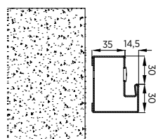
Rys. 7. Ościeżnica wewnętrzna
