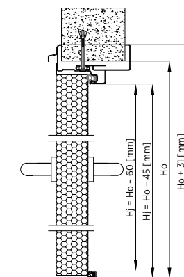
Rys. 60. Montaż do muru drzwi jednoskrzydłowych – ościeżnica obejmująca z przekładką termiczną – przekrój pionowy
