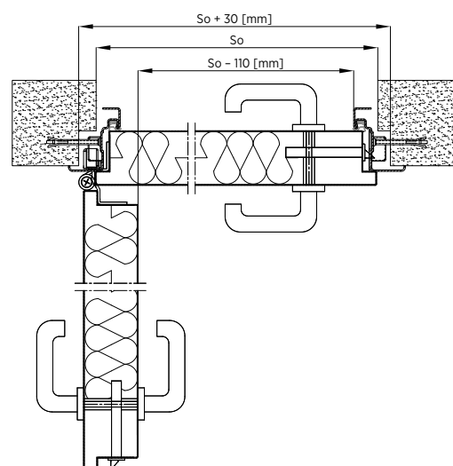
Rys. 46. Montaż do muru drzwi jednoskrzydłowych płaszczonek ECO TECH z ościeżnicą narożną bez przekładki termicznej – przekrój poziomy
