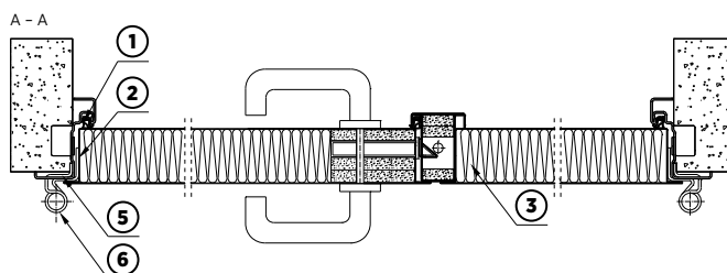
Rys. 6. Przekrój poziomy drzwi stalowych dwuskrzydłowych płaszczowych przeciwpożarowych z ościeżnicą narożną
