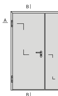
Rys. 4. Drzwi stalowe dwuskrzydłowe płaszczowe przeciwpożarowe
