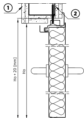
Rys. 41. Montaż do konstrukcji stalowej drzwi dwuskrzydłowych z ościeżnicą narożną – przekrój pionowy
