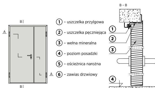
Rys. 75. Drzwi stalowe dwuskrzydłowe płaszczyne przeciwpożarowe wielkogabarytowe
