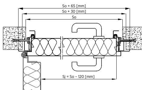
Rys. 54. Montaż do muru drzwi jednostronnych – ościeżnica narożna z przelączką termiczną – przekrój poziomy
