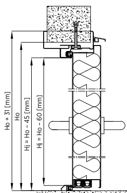
Rys. 57. Montaż do muru drzwi jednoskrzydłowych - ościeżnica obejmująca z przekładką - przekrój pionowy
