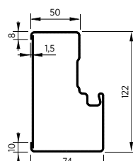
Rys. 54. Ościeżnica wewnętrzna
