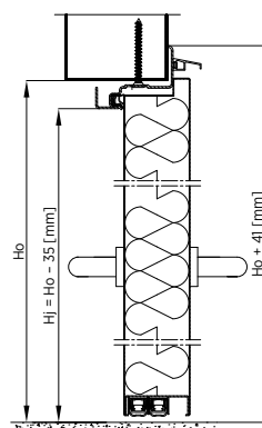
Rys. 53. Montaż do konstrukcji stalowej drzwi jednostronnych płaszczowych ECO TECH z ościeżnicą narożną bez przelączki termicznej – przekrój pionowy
