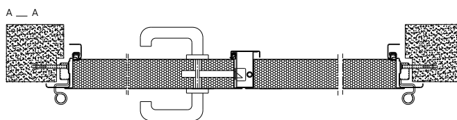
Rys. 6. Przekrój poziomy drzwi stalowych dwuskrzydłowych pełnych płaszczonek ECO z ościeżnicą na wysokości zamka
