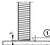
Rys. 60. Szczelina dolna drzwi bez progu ① – poziom posadzki
