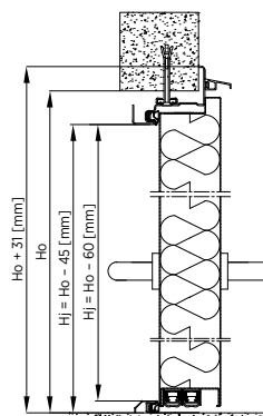
Rys. 55. Montaż do muru drzwi jednostronnych – ościeżnica narożna z przelączką termiczną – przekrój pionowy
