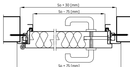
Rys. 52. Montaż do konstrukcji stalowej drzwi jednostronnych płaszczowych ECO TECH z ościeżnicą narożną bez przelączki termicznej – przekrój poziomy
