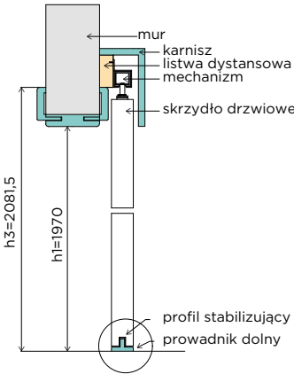
OPASKA 100 mm H1=1970 mm
