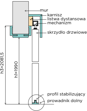
OPASKA 80 mm H1=1990 mm
