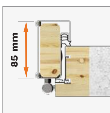
Ościeżnica DUOTHERM 75
