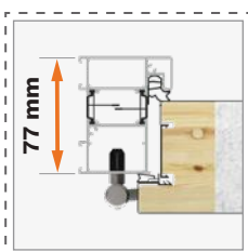
Ościeżnica ALUTHERM 75*
