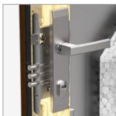
Zamek główny ryglowy
