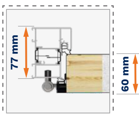
Ościeżnica ALUTHERM 60*
