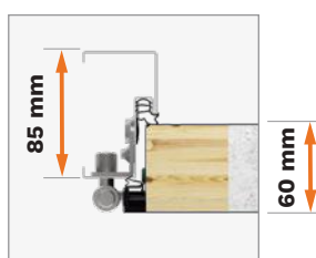
Ościeżnica PERFOTHERM 60
