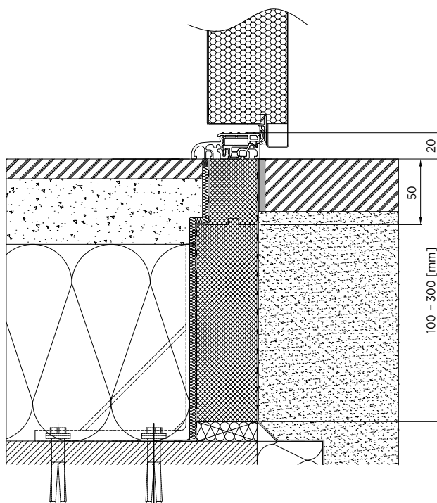
Rys. 31. Montaż progu aluminiowo-tworzywowego 52 [mm] z zastosowaniem profilu podprogowego z kątownikiem wzmacniającym - możliwość zamawiania do 300 [mm]
