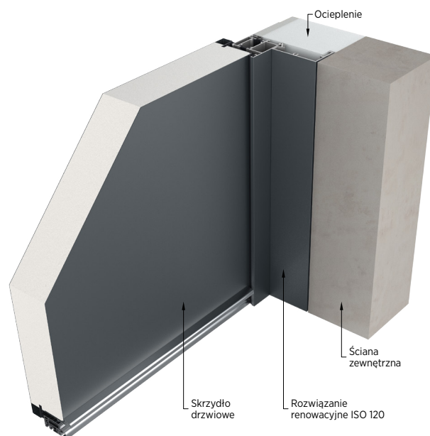
Rys. 44. Rozwiązanie renowacyjne ISO 120 z kątownikiem 60 [mm] – widok od zewnątrz
