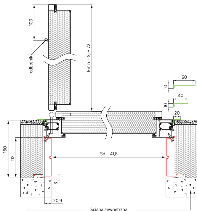
Rys. 43. Renowacja ISO 160 – przekrój poziomy – otwierane do wewnątrz – Drzwi NOBE
