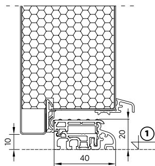
Rys. 32. Przekrój progów aluminiowo-tworzywowego 40 [mm] drzwi otwieranych do wewnątrz – rozwiązanie standardowe
