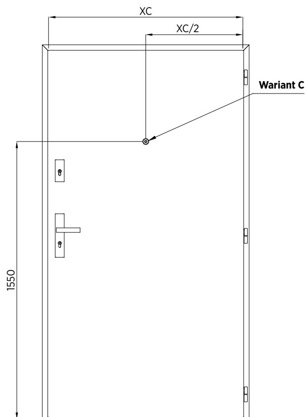
WARIANT C – wizjer w pionowej osi symetrii skrzydła
