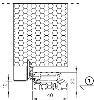
Rys. 26. Przekrój progu aluminiowo-tworzywowego 40 [mm] - rozwiązanie standardowe
