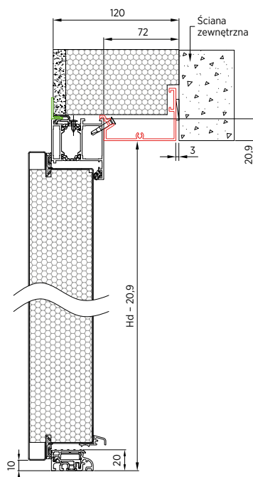
Rys. 40. Renowacja ISO 120 – przekrój pionowy – otwierane do wewnątrz – Drzwi NOBE
