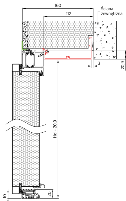
Rys. 42. Renowacja ISO 160 – przekrój pionowy – otwierane do wewnątrz – Drzwi NOBE
