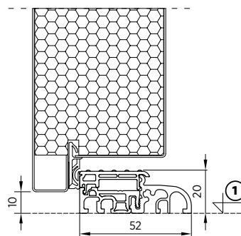
Rys. 29. Przekrój progu aluminiowo-tworzywowego 52 [mm] - rozwiązanie opcjonalne
