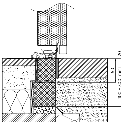
Rys. 30. Montaż progu aluminiowo-tworzywowego 52 [mm] z zastosowaniem profilu podprogowego
