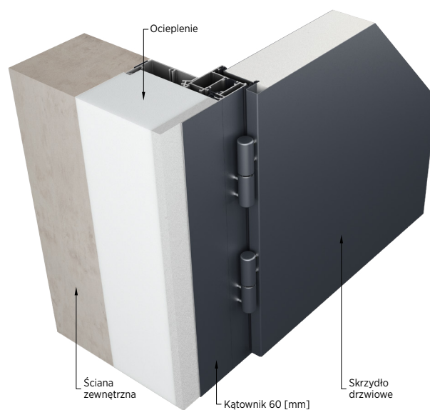
Rys. 45. Rozwiązanie renowacyjne ISO 120 z kątownikiem 60 [mm] – widok od wewnątrz
