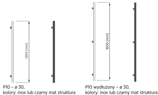
Rys. 19. Wzory uchwytów P10 do montażu na skraju skrzydła
