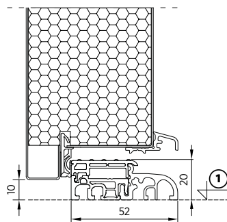
Rys. 33. Przekrój progów aluminiowo-tworzywowego 52 [mm] drzwi otwieranych do wewnątrz – rozwiązanie opcjonalne
