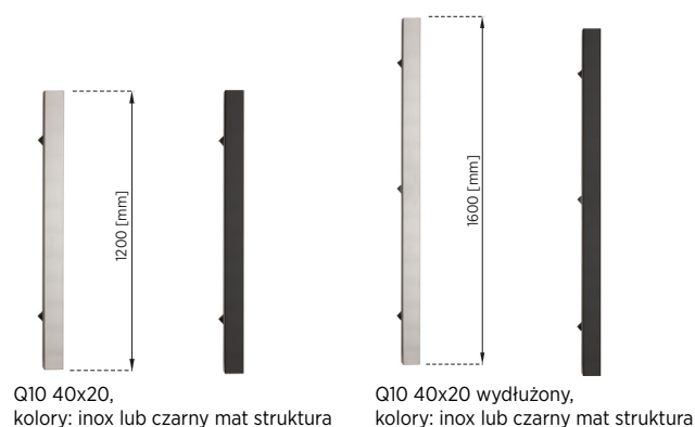
Rys. 20. Wzory uchwytów Q10 40x20 do montażu w wypełnieniu skrzydła
