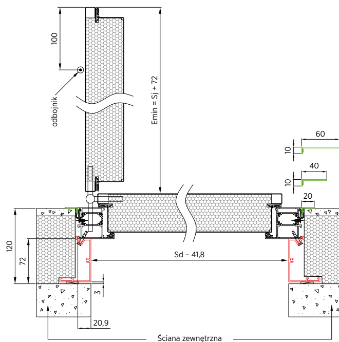
Rys. 41. Renowacja ISO 120 – przekrój poziomy – otwierane do wewnątrz – Drzwi NOBE
