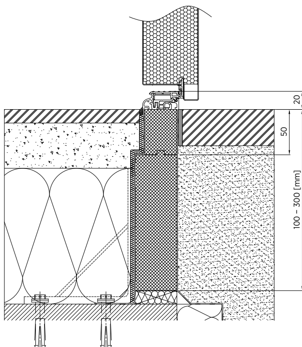
Rys. 28. Montaż progu aluminiowo-tworzywowego 40 [mm] z zastosowaniem profilu podprogowego z kątownikiem wzmacniającym - możliwość zamawiania do 300 [mm]
