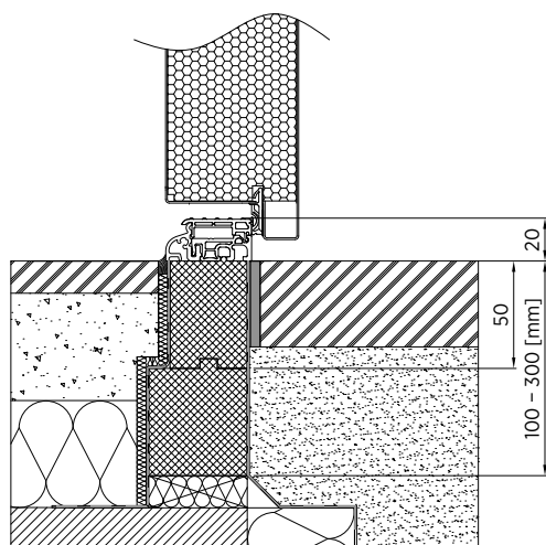
Rys. 27. Montaż progu aluminiowo-tworzywowego 40 [mm] z zastosowaniem profilu podprogowego
