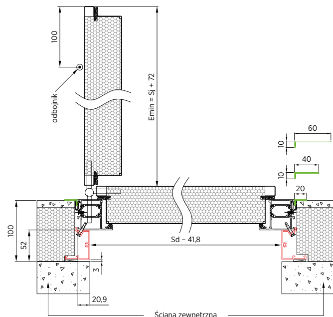
Rys. 39. Renowacja ISO 100 – przekrój poziomy – otwierane do wewnątrz – Drzwi NOBE
