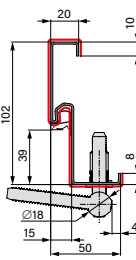
OŚCIEŻNICA STALOWA NAROŻNA
