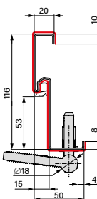
OŚCIEŻNICA STALOWA NAROŻNA
