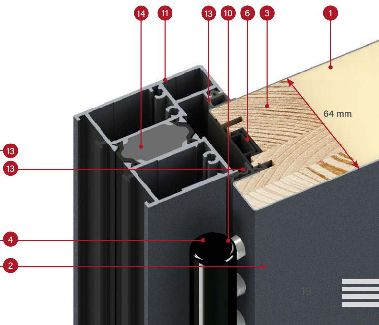
przekrój ościeżnicy stalowej dla skrzydła THERMO 64
