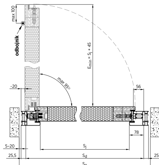
Rys. 73. Montaż w otworze – przekrój poziomy – drzwi NOVA z zawiasami ukrytymi i poszerzenia z obu stron – drzwi otwierane do wewnątrz
