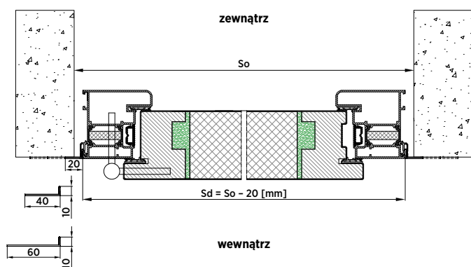
Rys. 81. Montaż w otworze z kątownikiem renowacyjnym od wewnątrz – przekrój poziomy – drzwi NOVA
