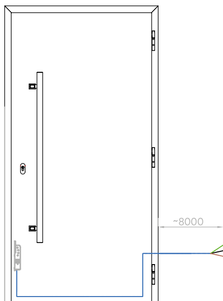
Rys. 38. Zamek trzypunktowy Autotronic – schemat wyprowadzenia przewodu
