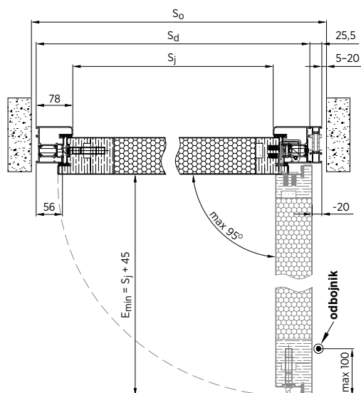
Rys. 70. Montaż w otworze – przekrój poziomy – drzwi NOVA z zawiasami ukrytymi i poszerzeniem z jednej strony – drzwi otwierane na zewnątrz
