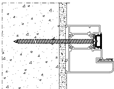
Rys. 76. Montaż bezpośredni za pomocą wkrętów hartowanych przez ościeżnicę (brak otworowania pod wkręty w profilu)
