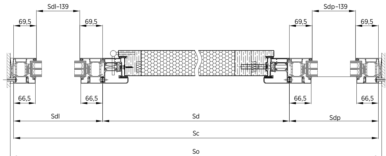
Rys. 91. Zależności wymiarowe dla doświetli bocznych
