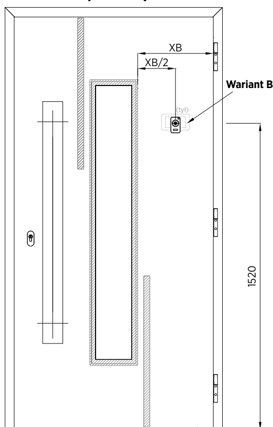
Rys. 68. Wizjer od strony zawiasów – przykład montażu dla wzoru 002
