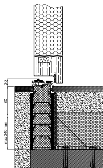
Rys. 59. Możliwość zastosowania dodatkowych profili o wysokości 30 [mm]. Maksymalna wysokość całego termo-poszerzenia to 320 [mm]. Powyżej wysokości 90 [mm] dodatkowego termo-poszerzenia należy go zamontować na kątownikach mocujących
