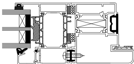
Rys. 78. Połączenie ościeżnicy z doświetlem / naświetlem (kierunek otwierania drzwi – na zewnątrz)
