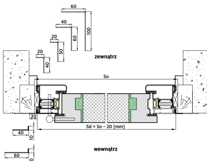
Rys. 85. Montaż w otworze z kątownikiem renowacyjnym od wewnątrz i od zewnątrz – przekrój poziomy – drzwi NOVA
