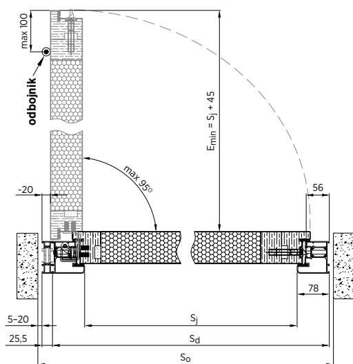
Rys. 71. Montaż w otworze – przekrój poziomy – drzwi NOVA z zawiasami ukrytymi i poszerzeniem z jednej strony – drzwi otwierane do wewnątrz
