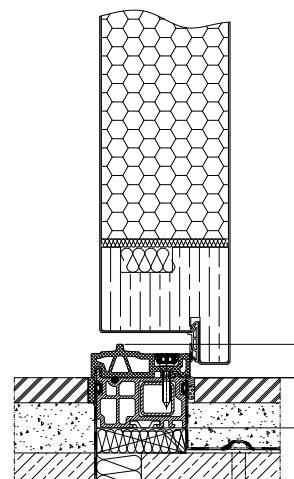
Rys. 54. Montaż progu z zastosowaniem profilu podprogowego o wysokości 30 [mm]
