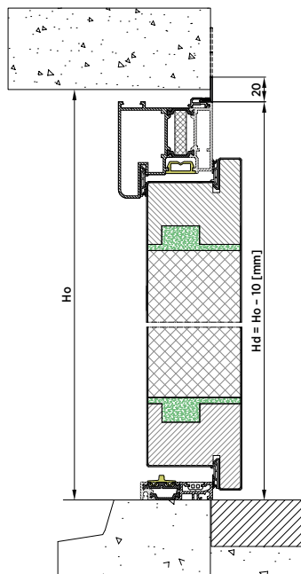
Rys. 80. Montaż w otworze z kątownikiem renowacyjnym od wewnątrz – przekrój pionowy – drzwi NOVA
