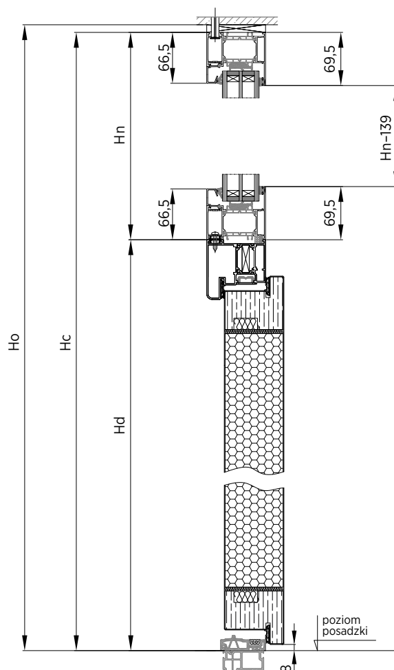
Rys. 92. Zależności wymiarowe dla naświetla górnego
