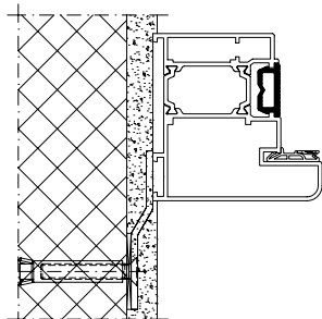
Rys. 74. Montaż za pomocą kotew stalowych (pośredni)
