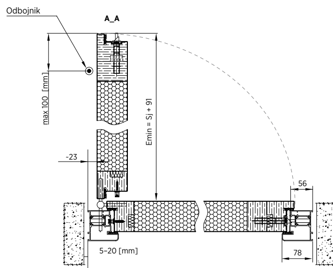
Rys. 7. Przekrój poziomy drzwi NOVA
