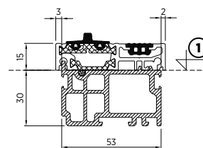
Rys. 53. Próg aluminiowy z zamontowanym profilem tworzywowym podprogowym
