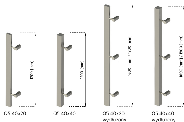
Rys. 31. Wzory uchwytów
