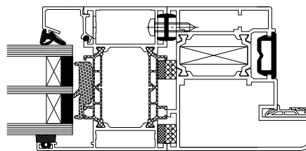
Rys. 79. Połączenie ościeżnicy z doświetlem / naświetlem (kierunek otwierania drzwi – do wewnątrz)
