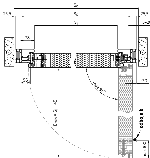
Rys. 72. Montaż w otworze – przekrój poziomy – drzwi NOVA z zawiasami ukrytymi i poszerzenia z obu stron – drzwi otwierane na zewnątrz
