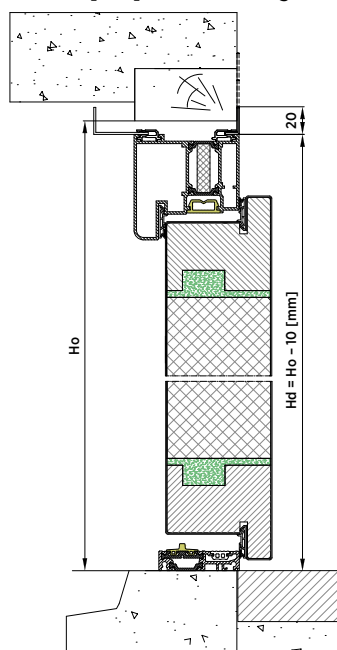
Rys. 84. Montaż w otworze z kątownikiem renowacyjnym od wewnątrz i od zewnątrz – przekrój pionowy – drzwi NOVA
