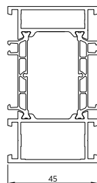
Rys. 88. Poszerzenie – szer. 45 [mm]
