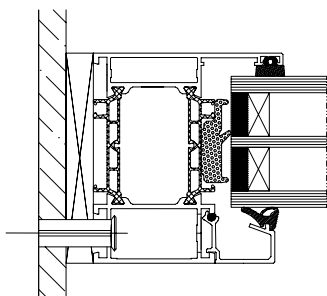
Rys. 77. Montaż bezpośredni ościeżnicy w przypadku doświetli / naświetli
