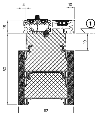
Rys. 56. Próg aluminiowy z zamontowanym termo-poszerzeniem Stropex 80 [mm]
