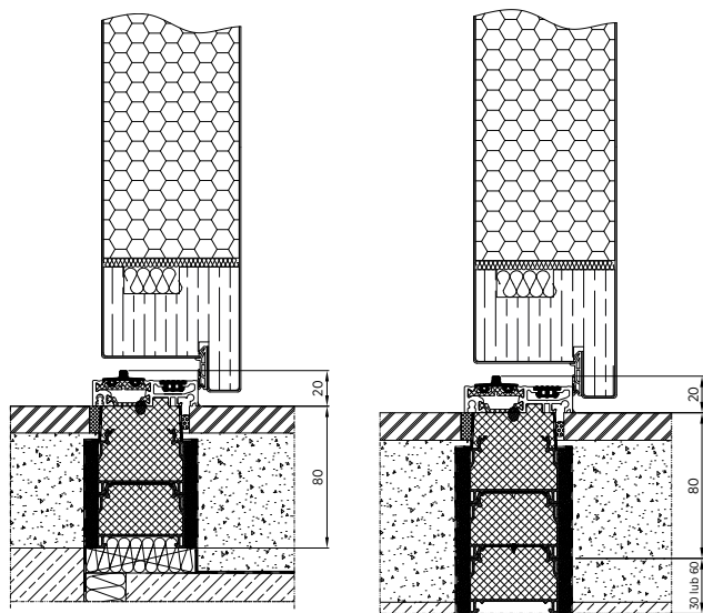
Rys. 57. Montaż progu z termo-poszerzeniem Stropex o wysokości 80 [mm]
