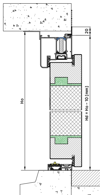
Rys. 82. Montaż w otworze z kątownikiem renowacyjnym od wewnątrz i od zewnątrz – przekrój pionowy – drzwi NOVA
