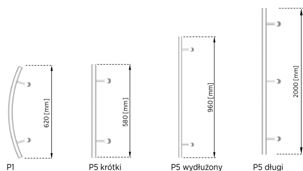
Rys. 31. Wzory uchwytów
