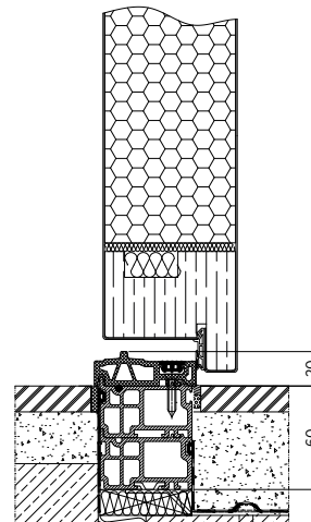
Rys. 55. Montaż progu z zastosowaniem dodatkowego profilu o wysokości 30 [mm] (maksymalna wysokość poszerzenia tego rozwiązania to 60 [mm])
