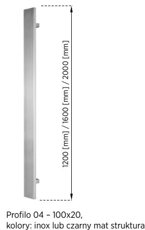
Rys. 32. Wzory uchwytów
