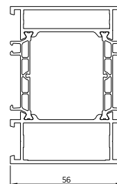
Rys. 89. Poszerzenie – szer. 56 [mm]
