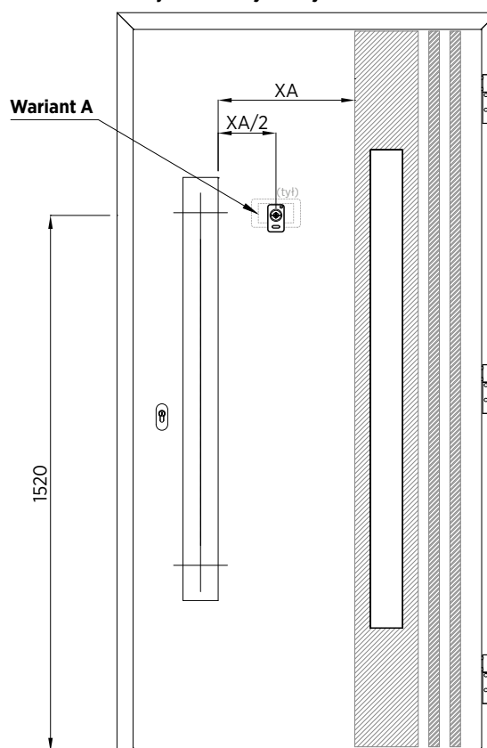
Rys. 67. Wizjer od strony uchwyty – przykład montażu dla wzoru 004
