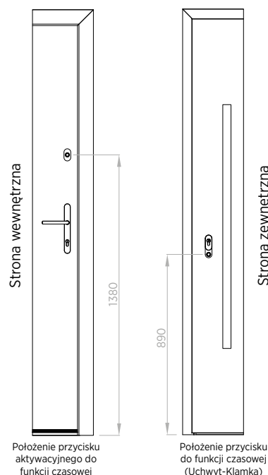
Rys. 39. Schemat położenia przycisków funkcji czasowej
