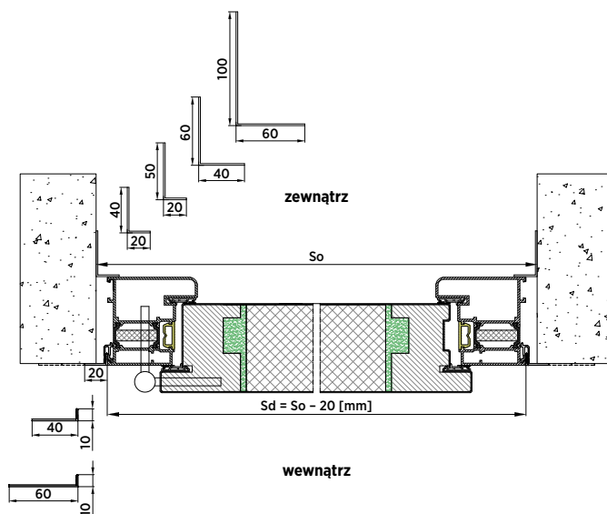
Rys. 83. Montaż w otworze z kątownikiem renowacyjnym od wewnątrz i od zewnątrz – przekrój poziomy – drzwi NOVA
