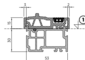
Rys. 52. Próg tworzywowy z zamontowanym profilem tworzywowym podprogowym
