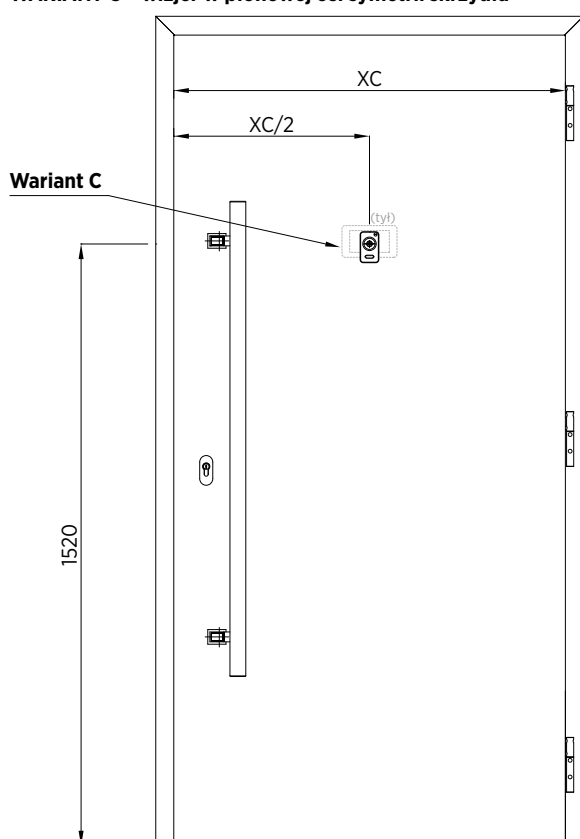
Rys. 69. Wizjer w pionowej osi symetrii skrzydła – przykład montażu dla wzoru 001
