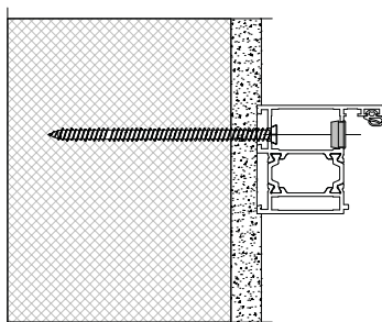
Rys. 51. Montaż za pomocą wkrętów hartowanych przez ościeżnicę (bezpośredni)
