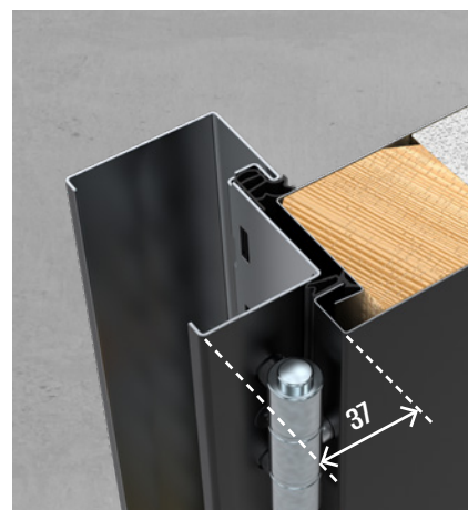
OŚCIEŻNICA PERFOTHERM 60 XL
