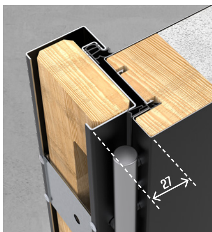
OŚCIEŻNICA DUOTHERM 75
