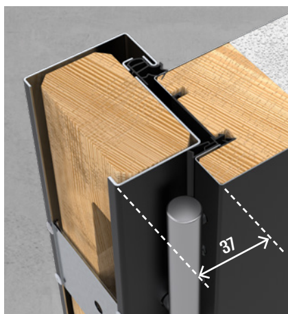
OŚCIEŻNICA DUOTHERM 75 XL
