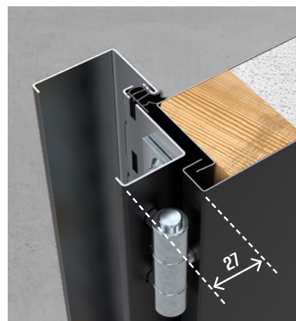
OŚCIEŻNICA PERFOTHERM 60
