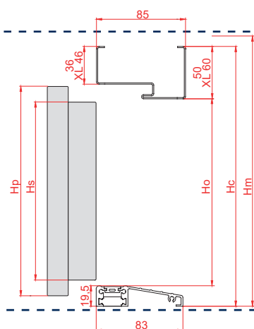
DUOTHERM 60 DUOTHERM 60 XL
