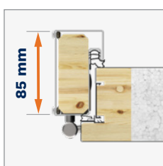
Ościeżnica DUOTHERM 75
