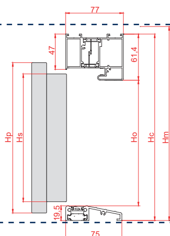
ALUTHERM 60
