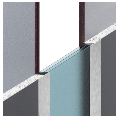
PAKIEŃ 3-SZYBOWY Z RAMKĄ XN
