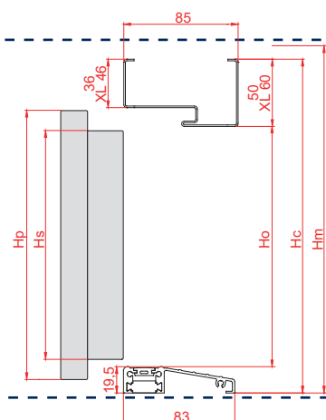
DUOTHERM 75 DUOTHERM 75 XL
