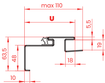
PROFIL OŚCIEŻNICY
