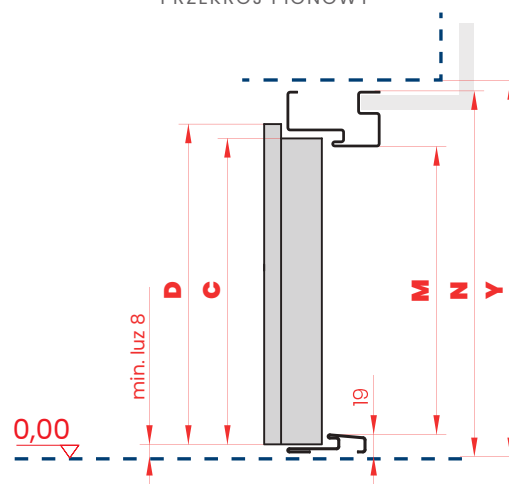
PRZEKRÓJ PIONOWY
