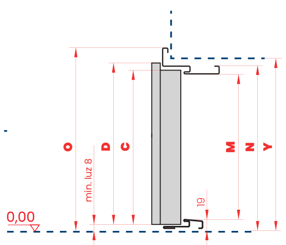
PRZEKRÓJ PIONOWY
