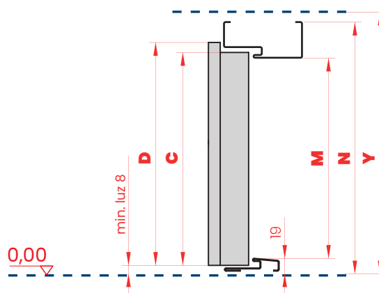
PRZEKRÓJ PIONOWY
