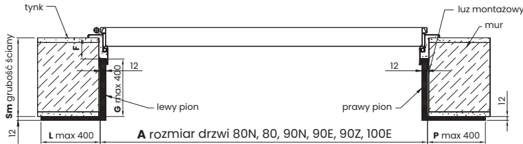
PRZEKRÓJ POZIOMY
