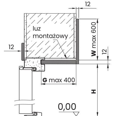
PRZEKRÓJ PIONOWY
