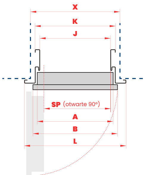
PRZEKRÓJ POZIOMY
