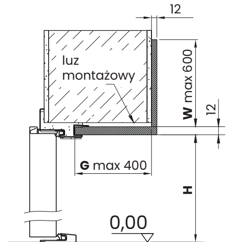
PRZEKRÓJ PIONOWY
