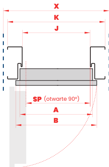
PRZEKRÓJ POZIOMY
