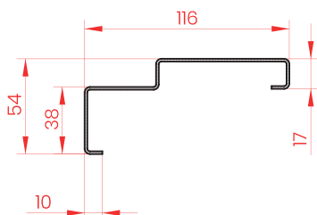
PROFIL OŚCIEŻNICY
