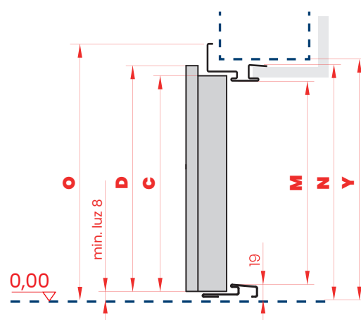
PRZEKRÓJ PIONOWY
