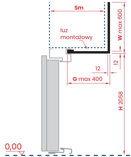
PRZEKRÓJ PIONOWY
