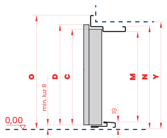
PRZEKRÓJ PIONOWY
