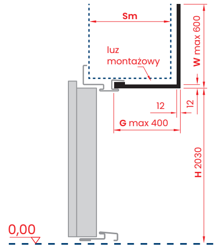
PRZEKRÓJ PIONOWY
