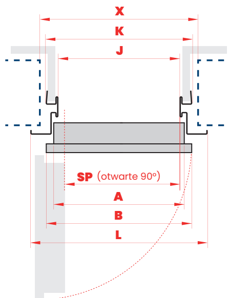
PRZEKRÓJ POZIOMY
