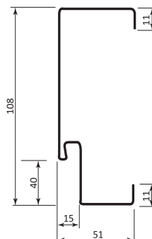
Ościeznica „11” EXPERT 64
