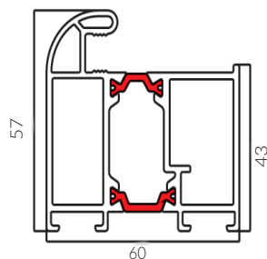
Ościeznica „TERMO do EXPERT 64”
